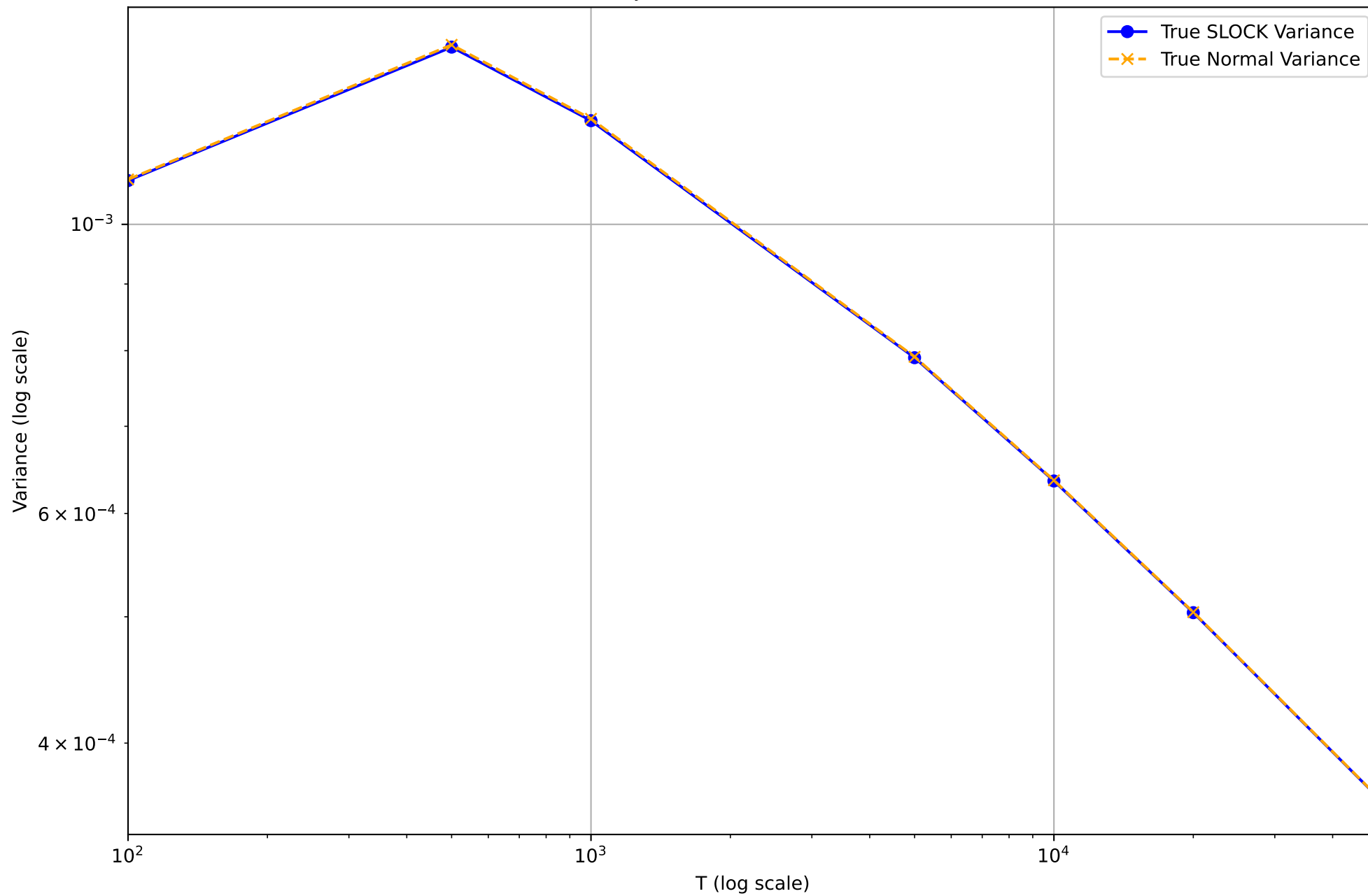
True Variance Trajectories (SLOCK vs Normal) eta=0.01
