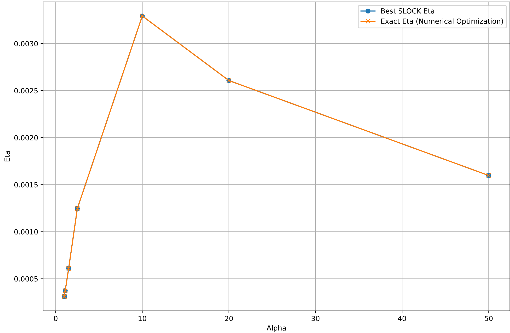
Comparison of Best SLOCK Eta vs Exact Eta (Numerical Optimization); T=100000, Delta=1
