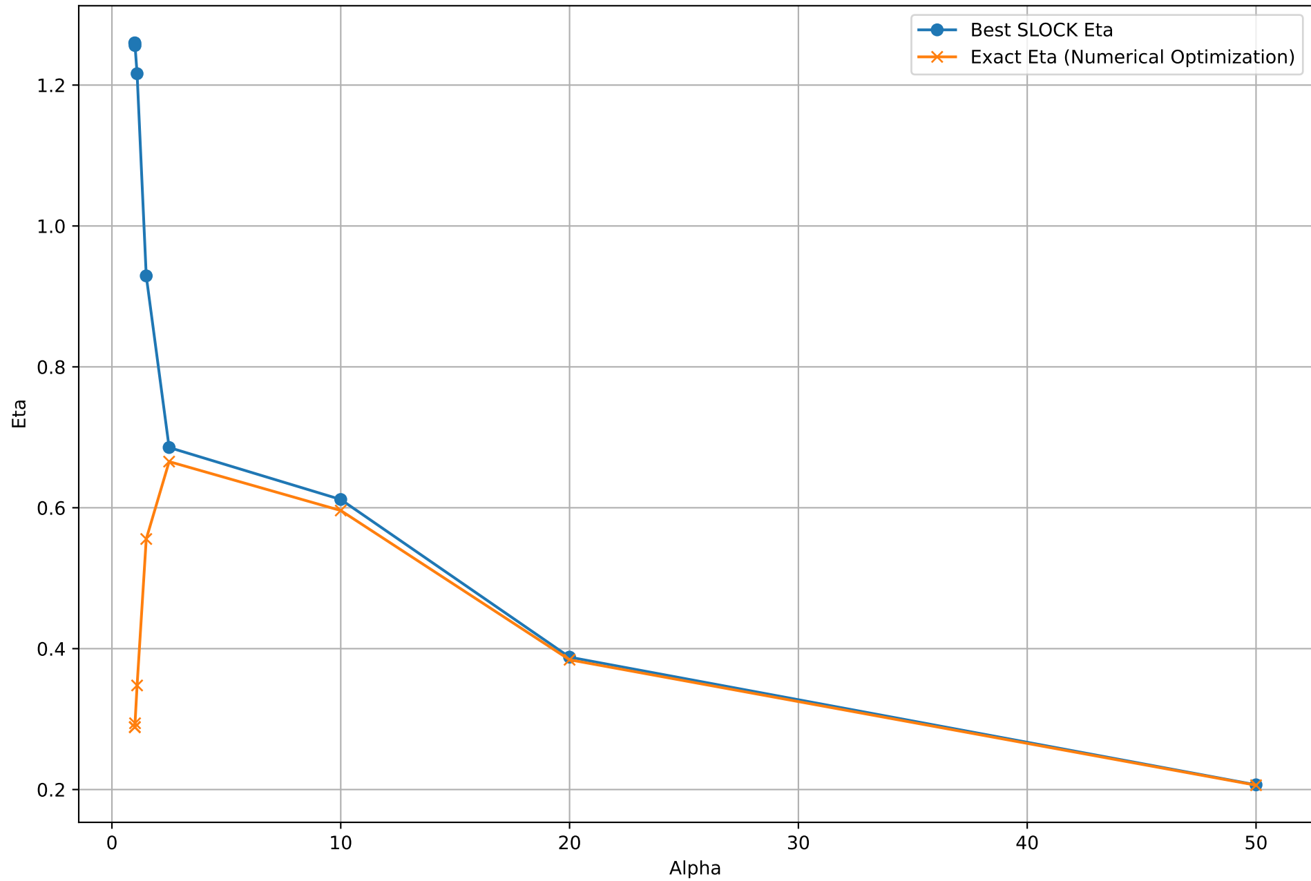
Comparison of Best SLOCK Eta vs Exact Eta (Numerical Optimization); T=1 , \Delta t=1
