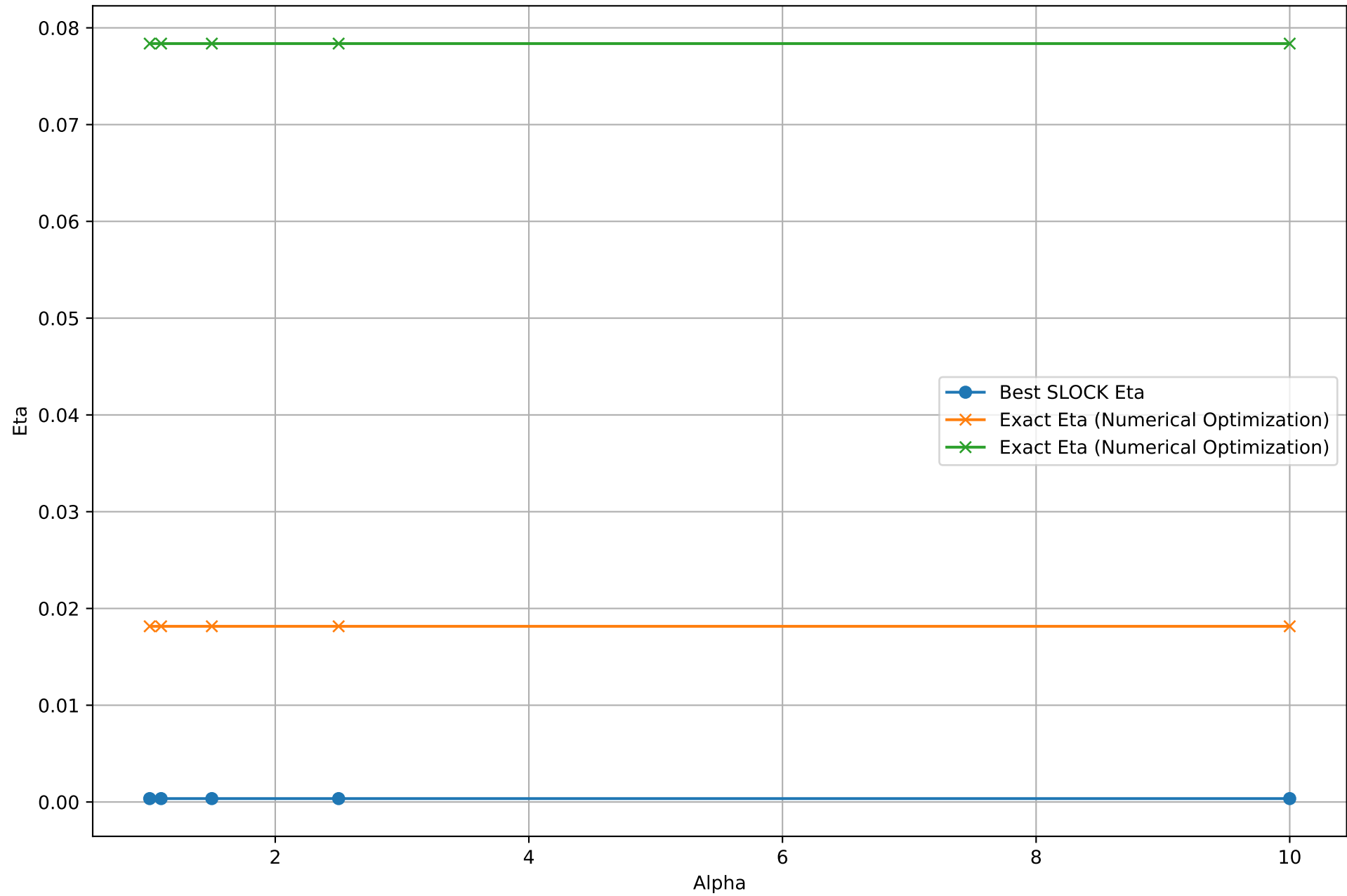
Comparison of Best SLOCK Eta vs Exact Eta (Numerical Optimization); T=50000, Delta=1
