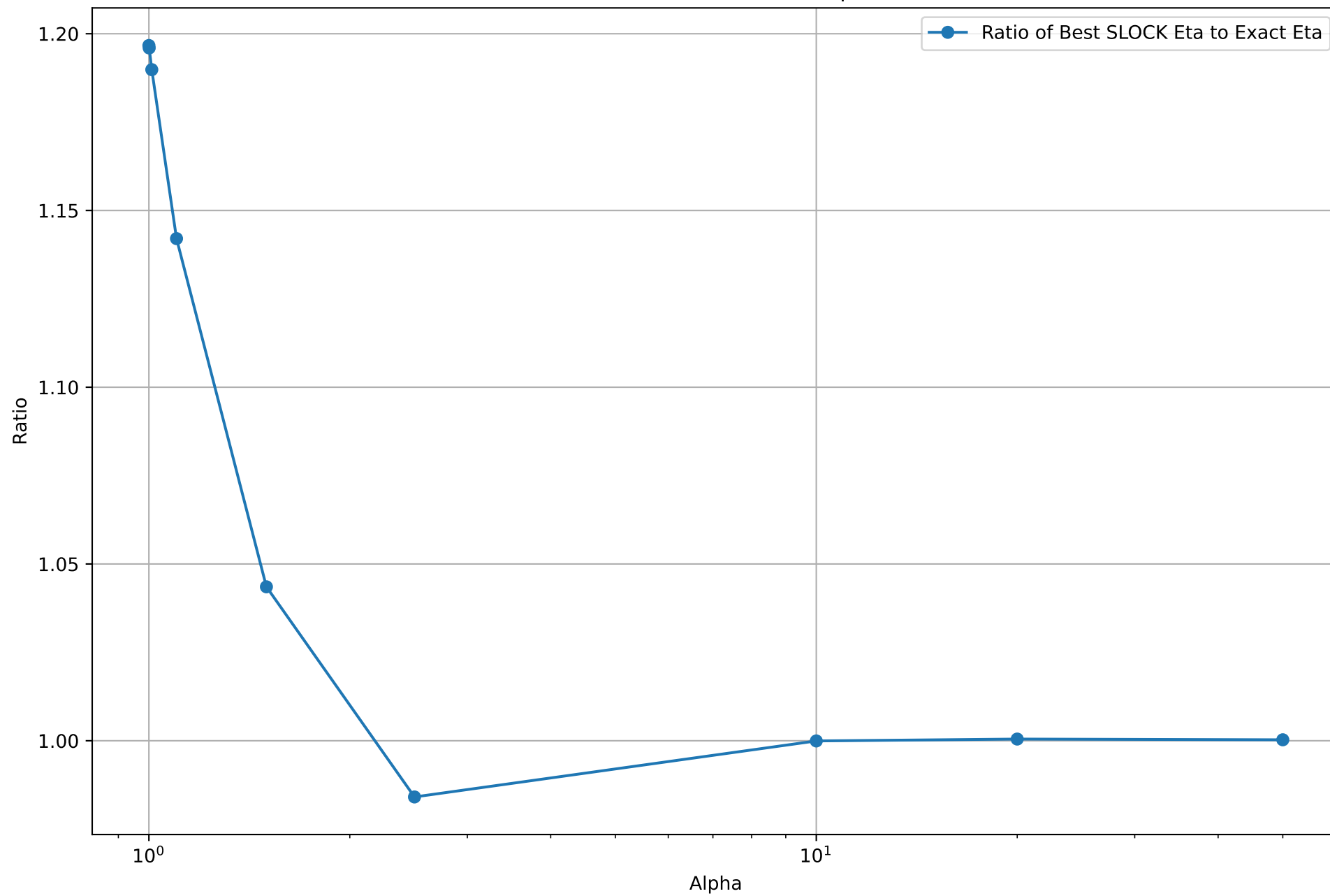
Ratio of Best SLOCK Eta to Exact Eta (Numerical Optimization); T=10, Delta=1
