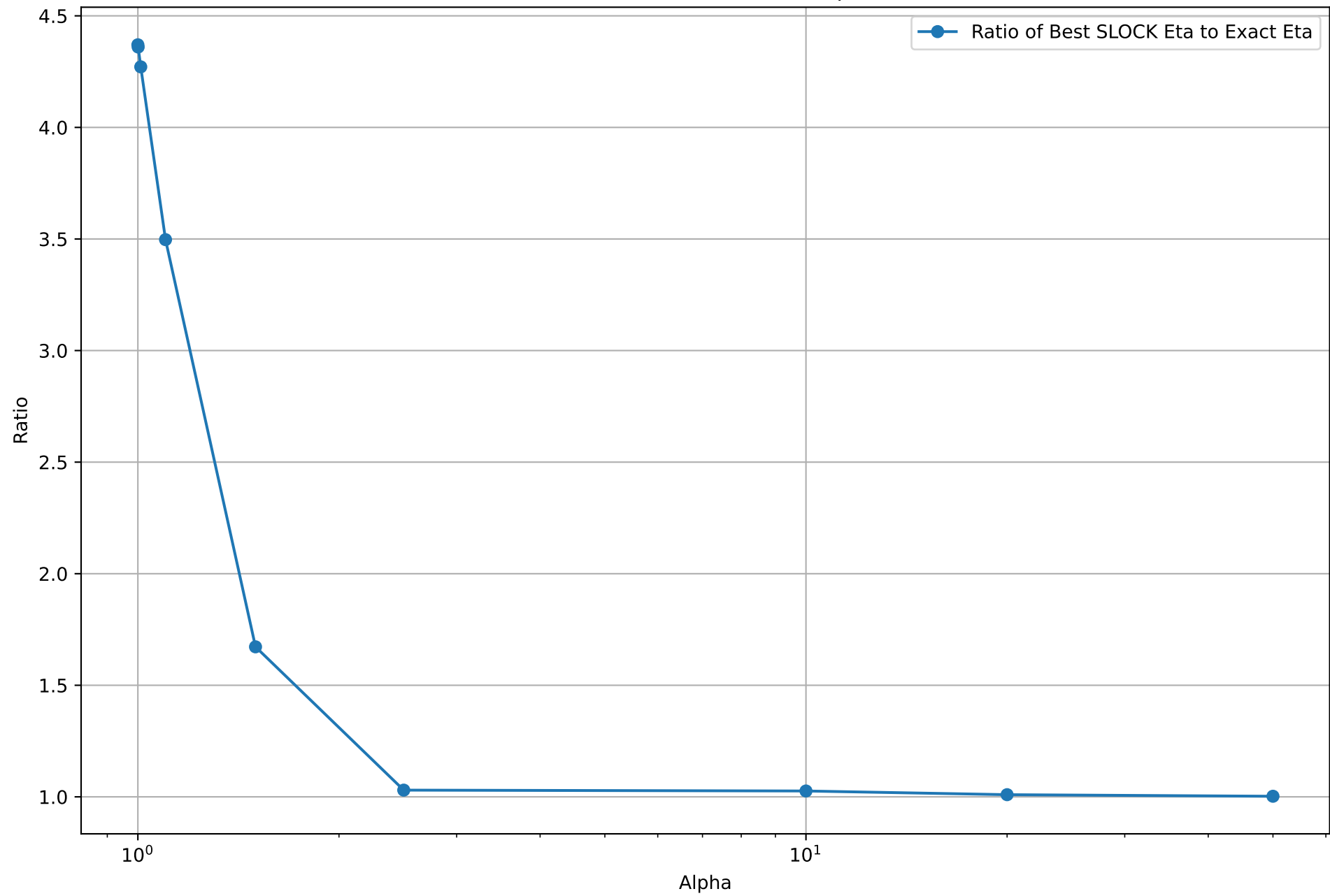
Ratio of Best SLOCK Eta to Exact Eta (Numerical Optimization); T=1, Delta=1
