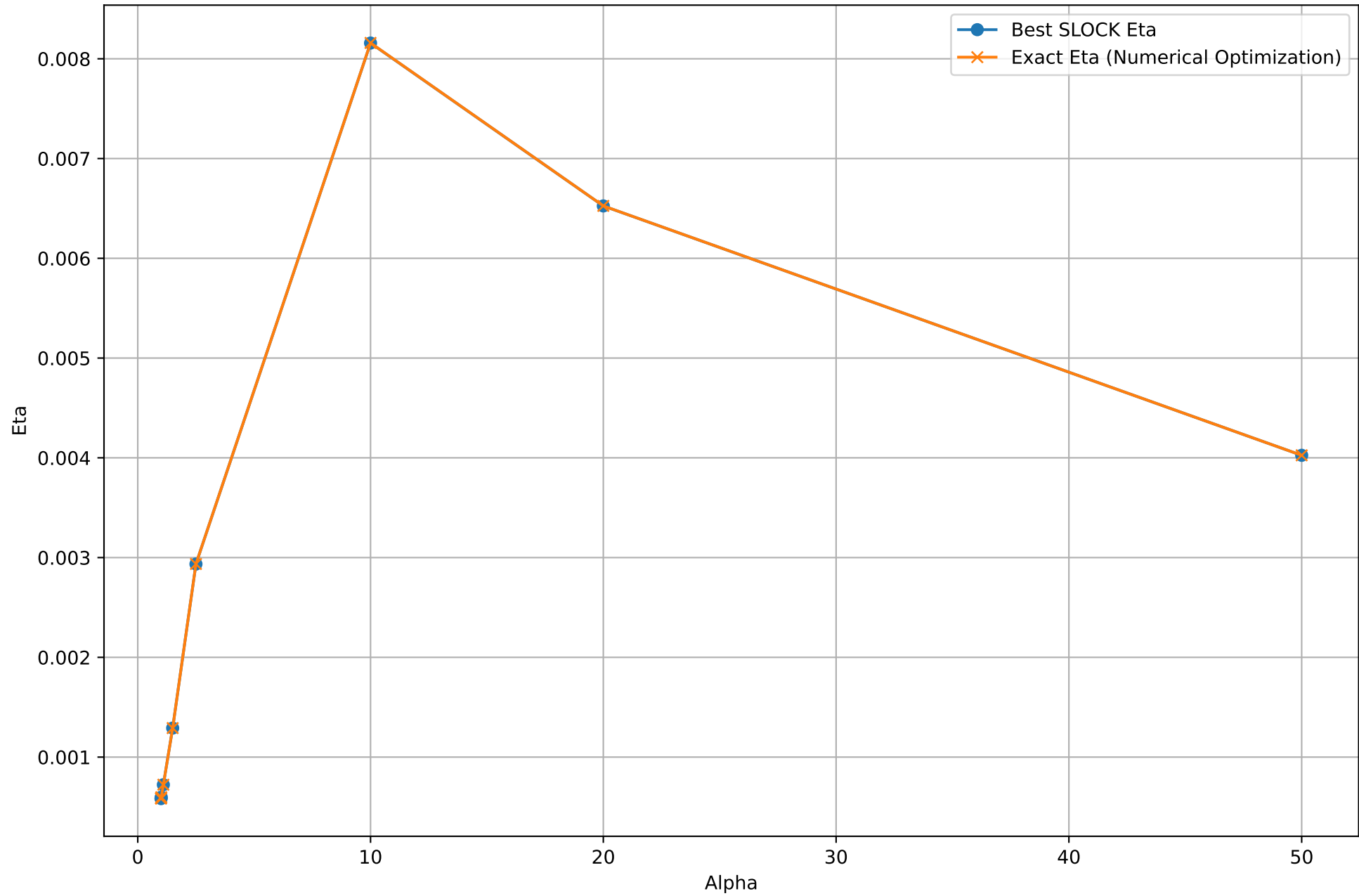
Comparison of Best SLOCK Eta vs Exact Eta (Numerical Optimization); T=100000, Delta=1
