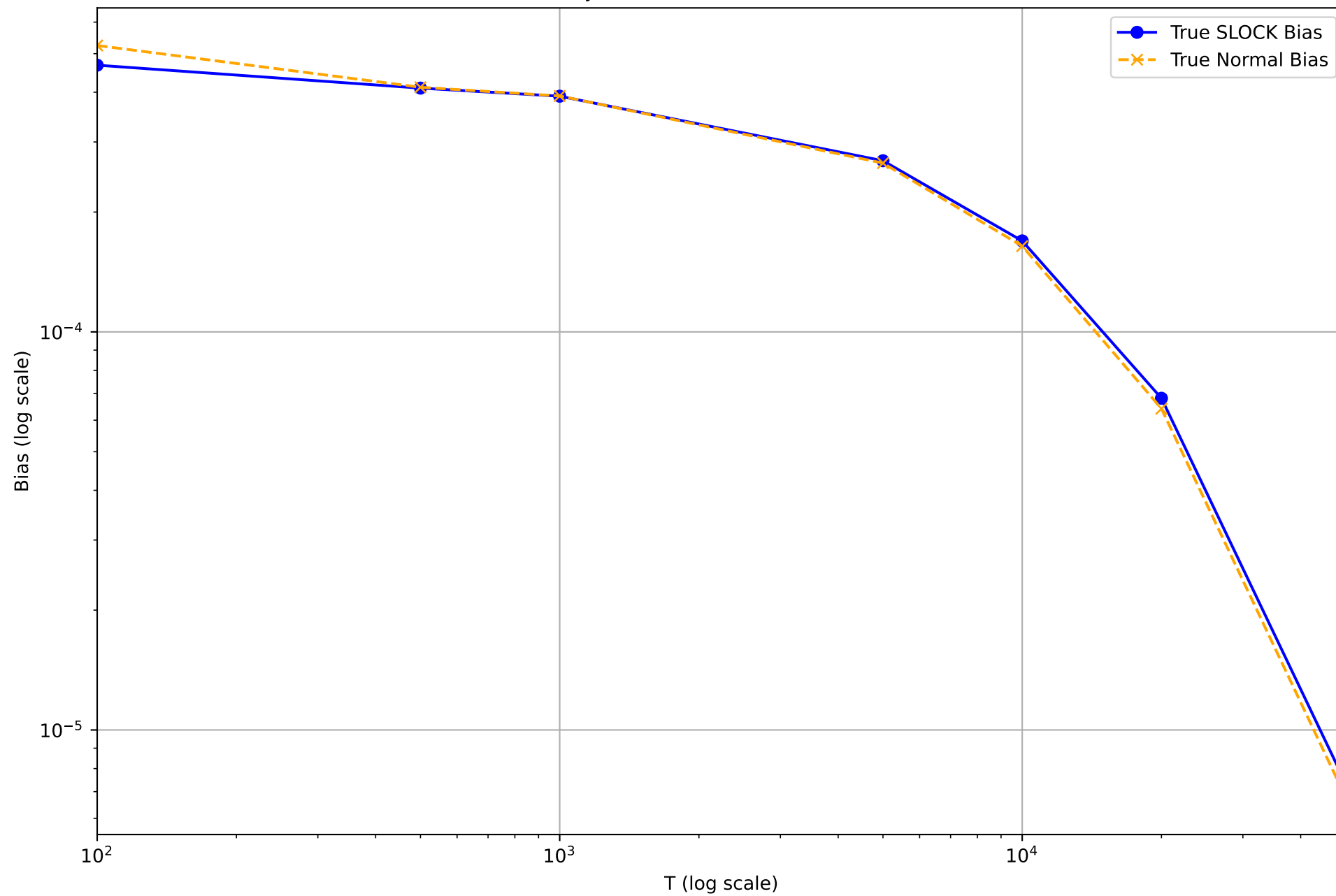
True Bias Trajectories (SLOCK vs Normal) eta=0.1
