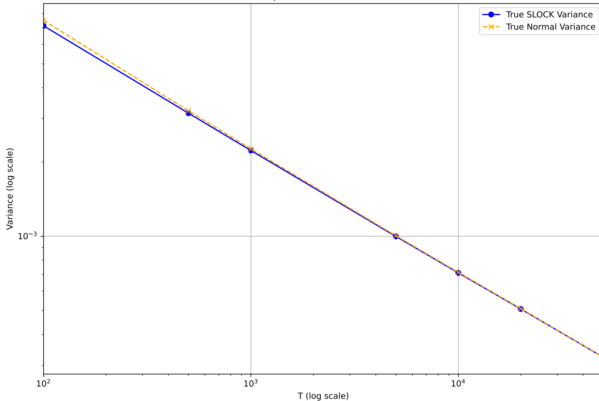
True Variance Trajectories (SLOCK vs Normal) eta=0.1
