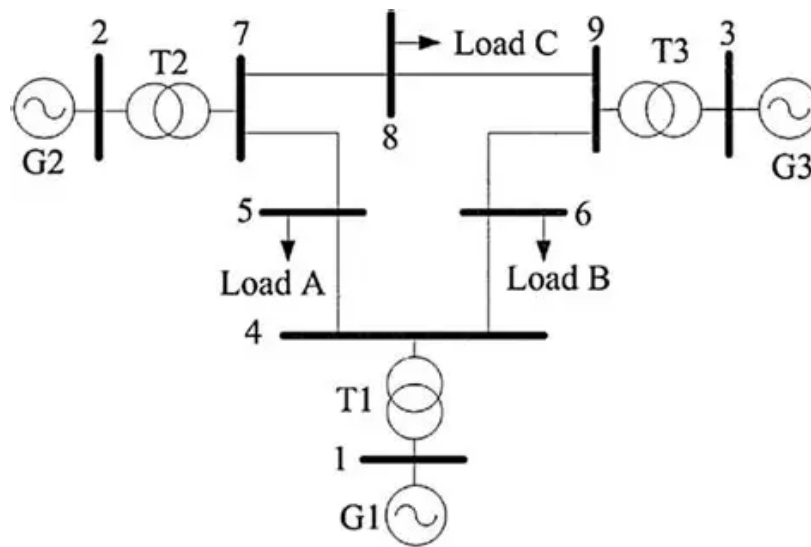
Gambar 2.11. Topologi Sistem Uji IEEE Nine-Bus [34]
