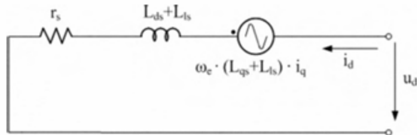
Gambar 2.9. D-Axis Equivalent Circuit PMSG dalam Kerangka Referensi Sinkron [30]
