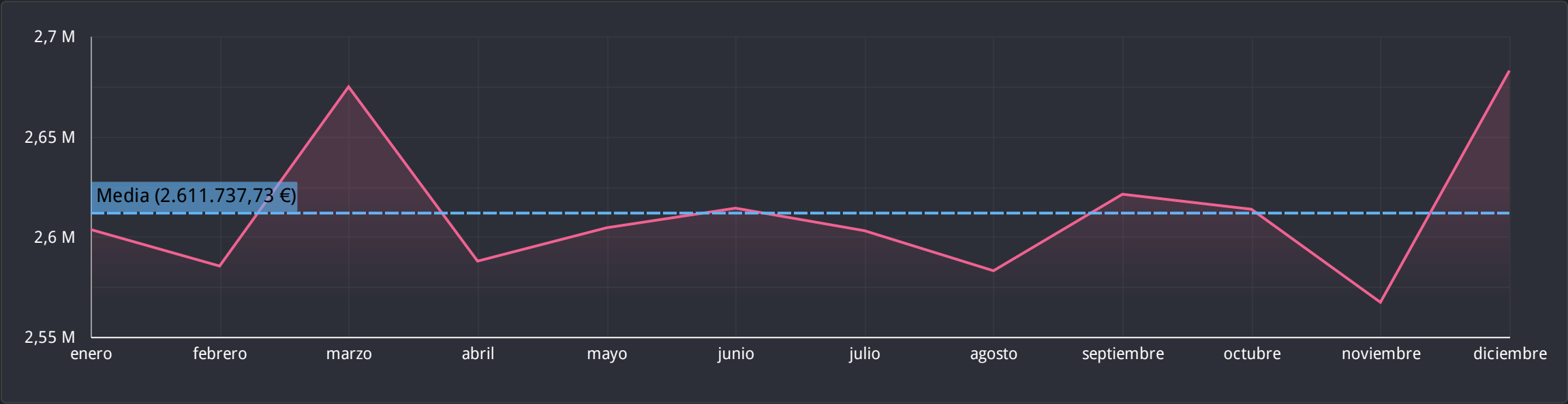
Total ganancias + IVA a lo largo del tiempo
