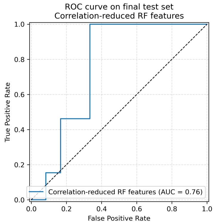
Figura 13: Curva ROC del modello Random Forest basato sul feature set ridotto in base alla correlazione.
