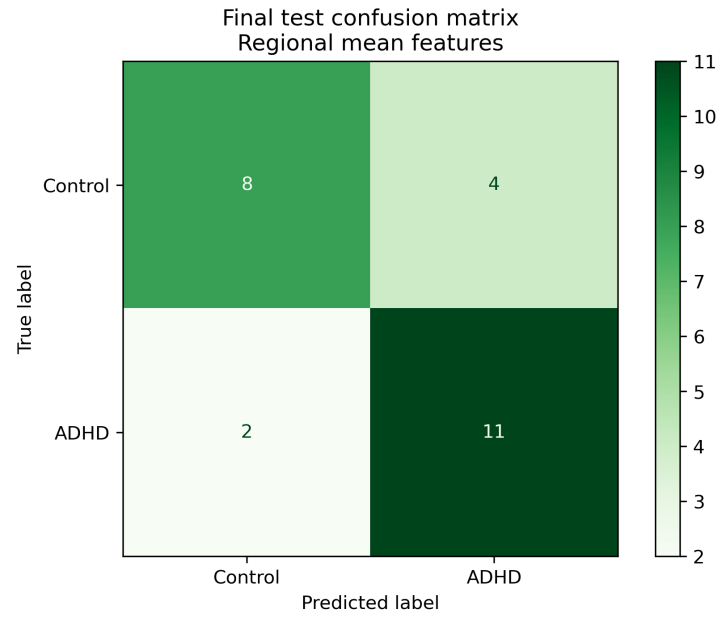
Figura 8: Confusion matrix del modello Random Forest finale valutato sul test set indipendente.
