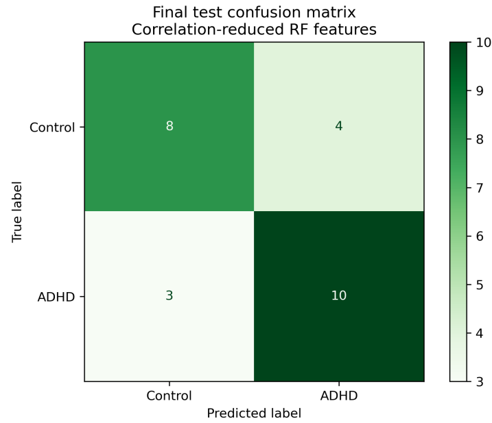
Figura 12: Confusion matrix del modello Random Forest basato sul feature set ridotto in base alla correlazione.
