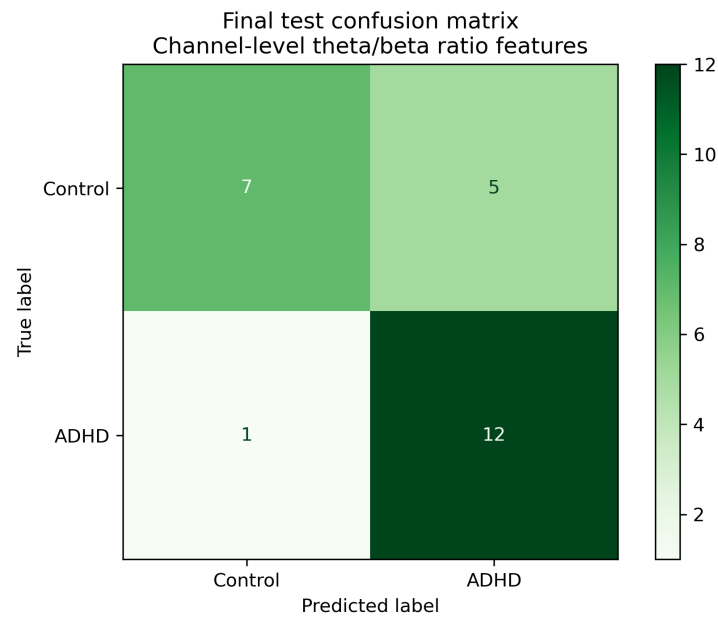
Figura 14: Confusion matrix del modello Random Forest basato sulle sole feature theta/beta ratio.
