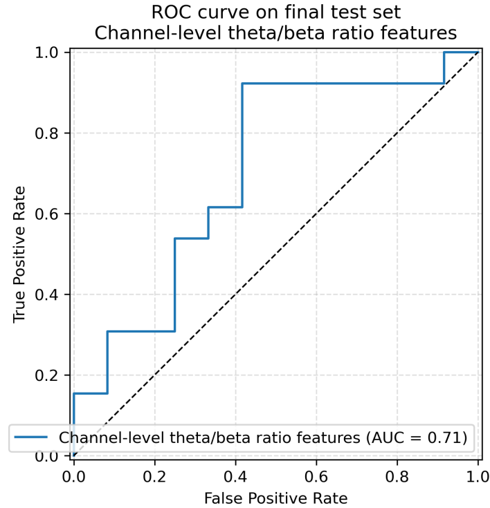
Figura 15: Curva ROC del modello Random Forest basato sulle sole feature theta/beta ratio.
