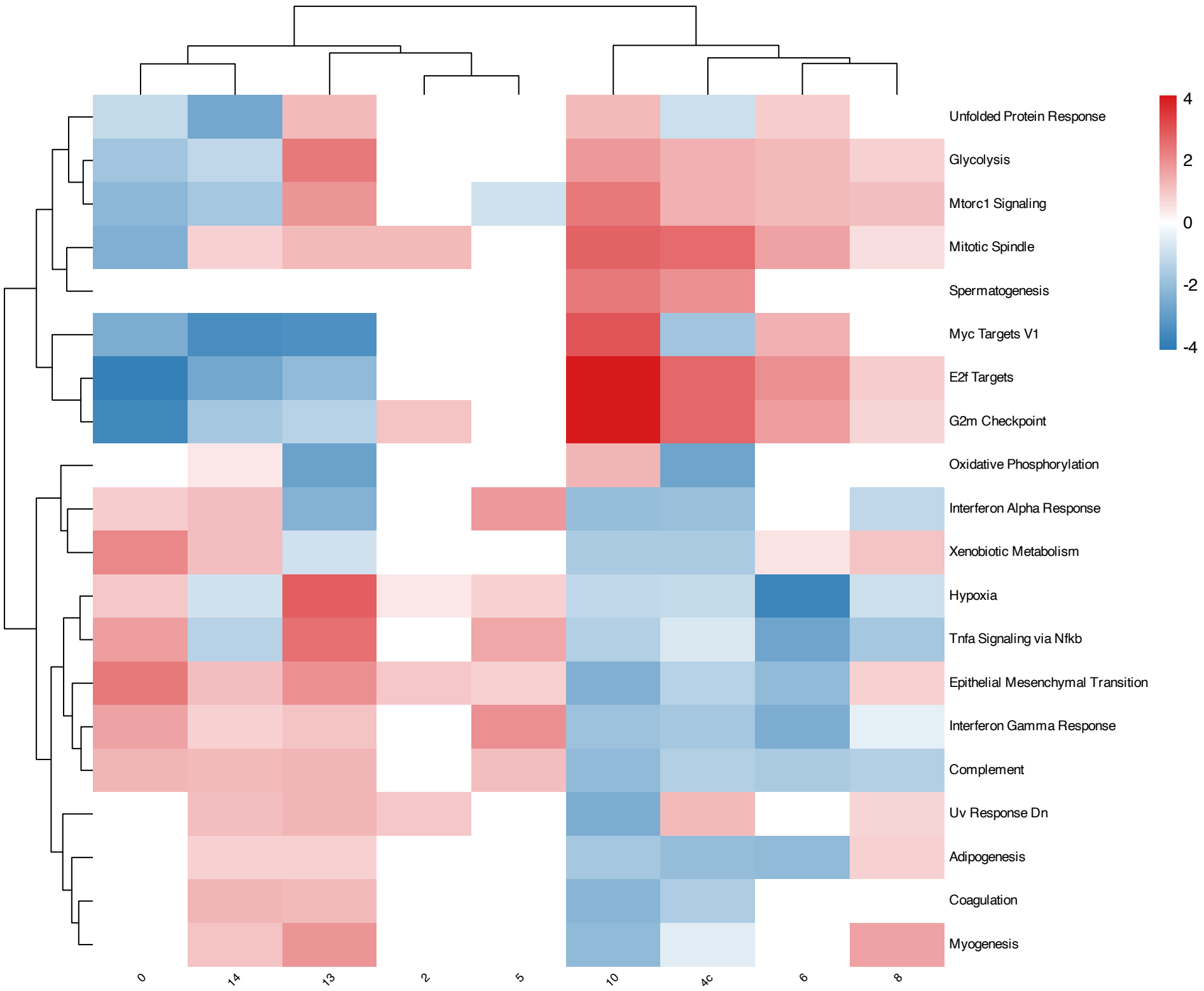
B Cluster Hallmark GSEA NES
