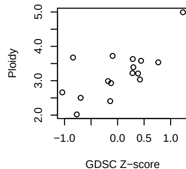
BLCA MG-132
