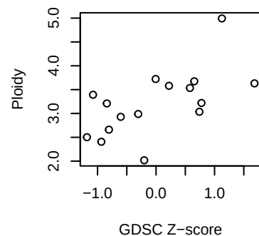
BLCA Pevonedistat
