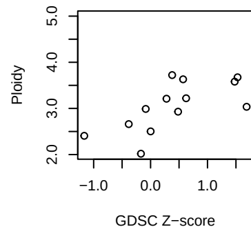
BLCA L-Oxonoreleagine
