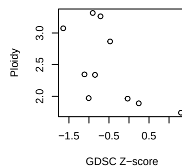
KIRC BEN
