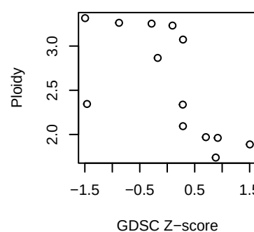
KIRC Afuresertib
