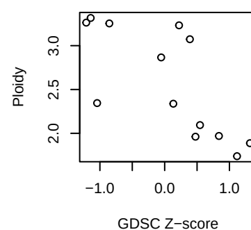
KIRC AZD5363
