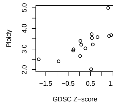
BLCA Talazoparib
