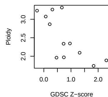
KIRC Entinostat
