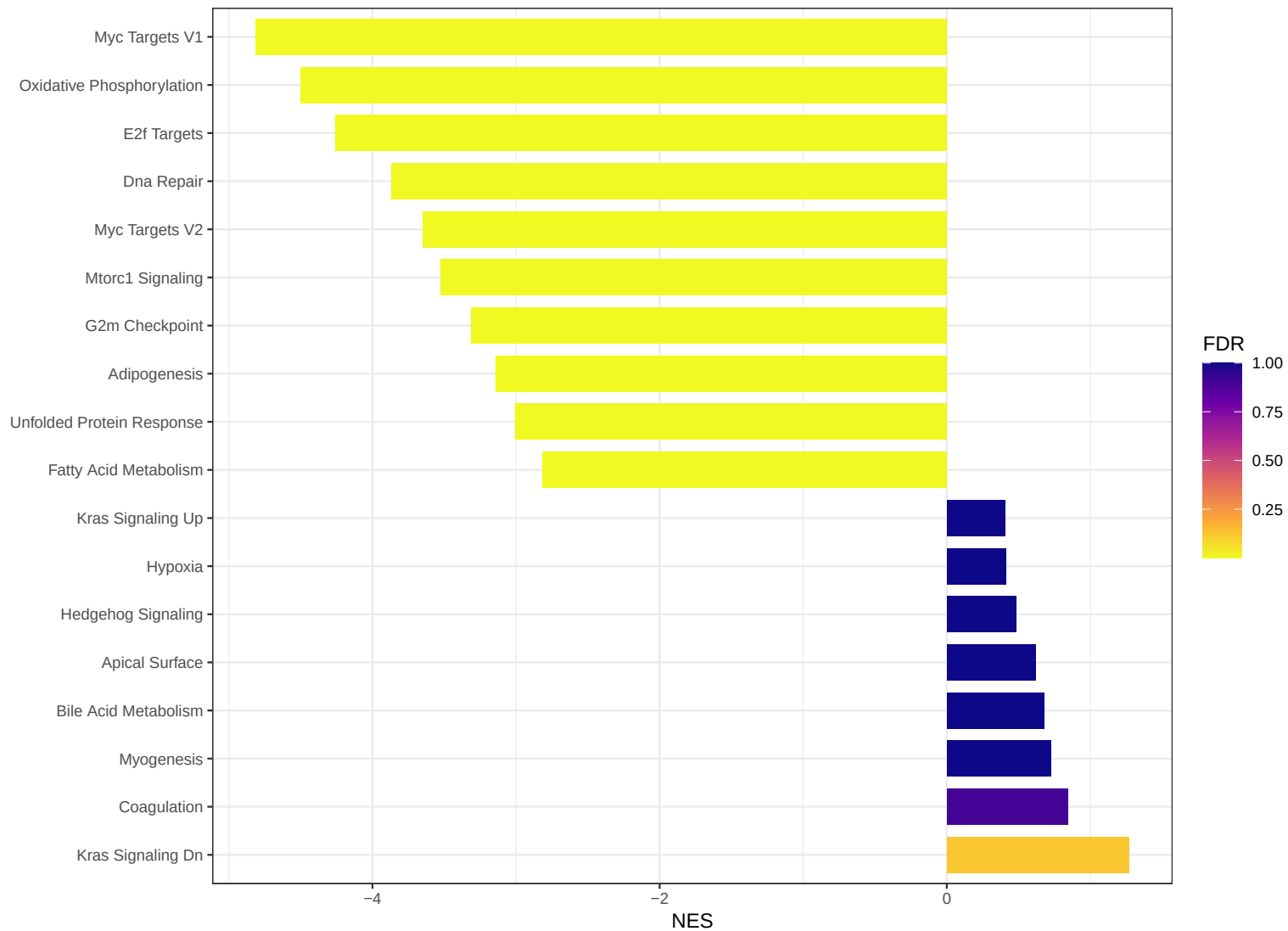
ETP_fixed_threshold_2_25: hallmark GSEA
