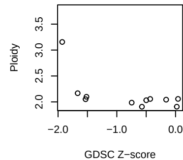
LAML Cytarabine
