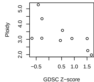
LGG EHT-1864
