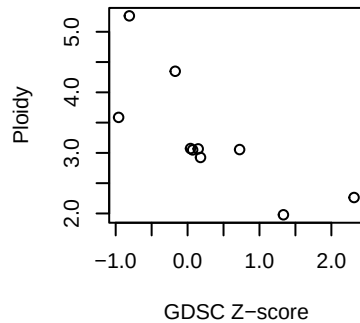
LGG MIRA-1
