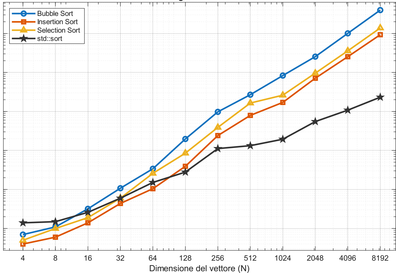
Confronto Algoritmi di Ordinamento
