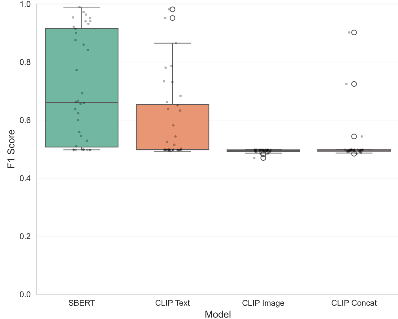
F1 Score Quartiles and Outliers
