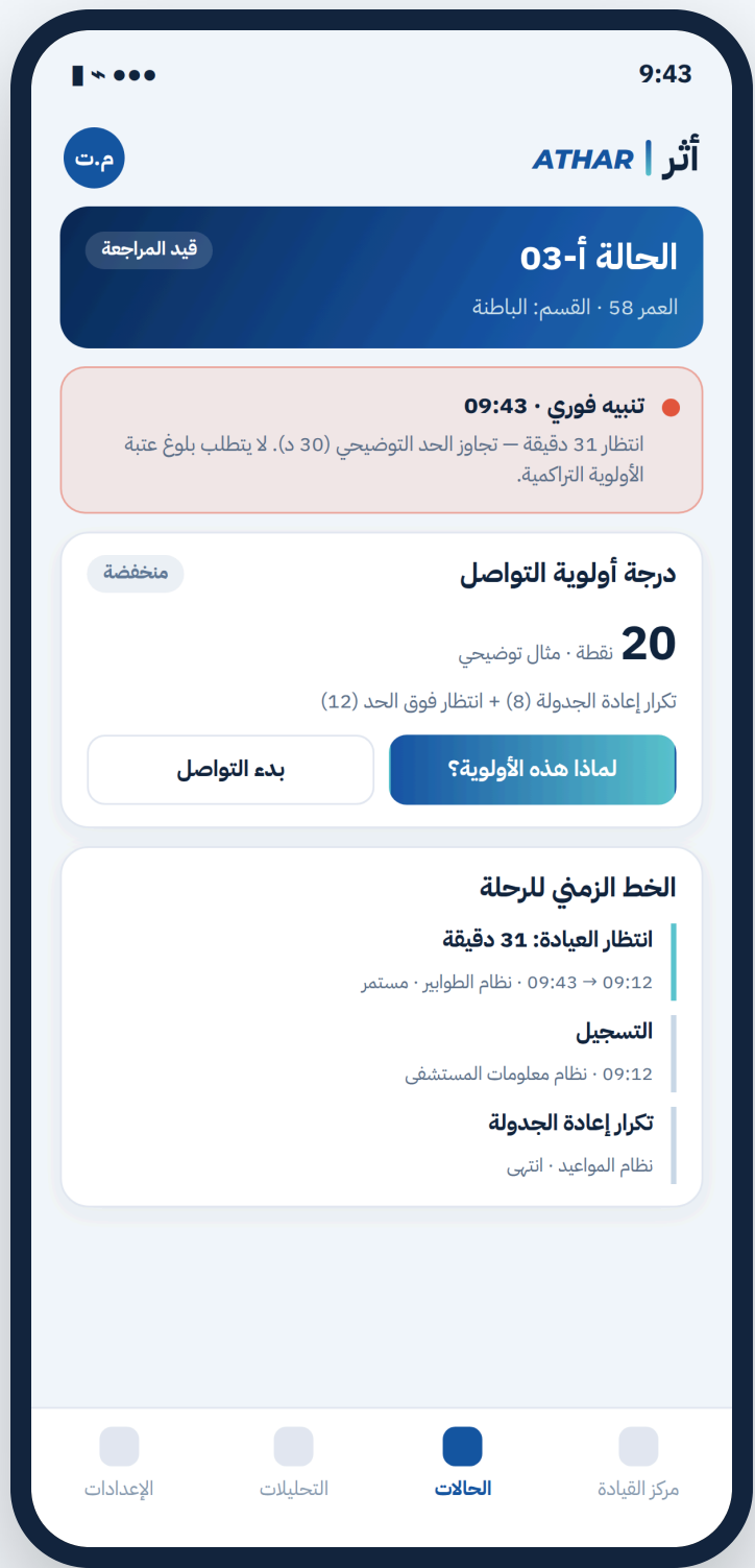
تفاصيل الحالة: التنبيه ثم الدرجة وزر «لماذا؟»
