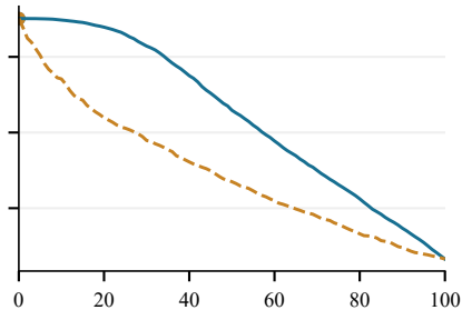
cub / GLSim
