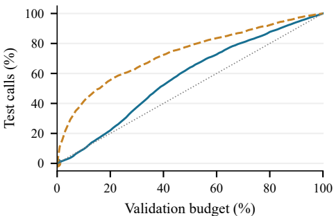
nlvr2 / BEiT3
