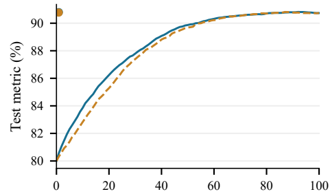
nlvr2 / BEiT3
