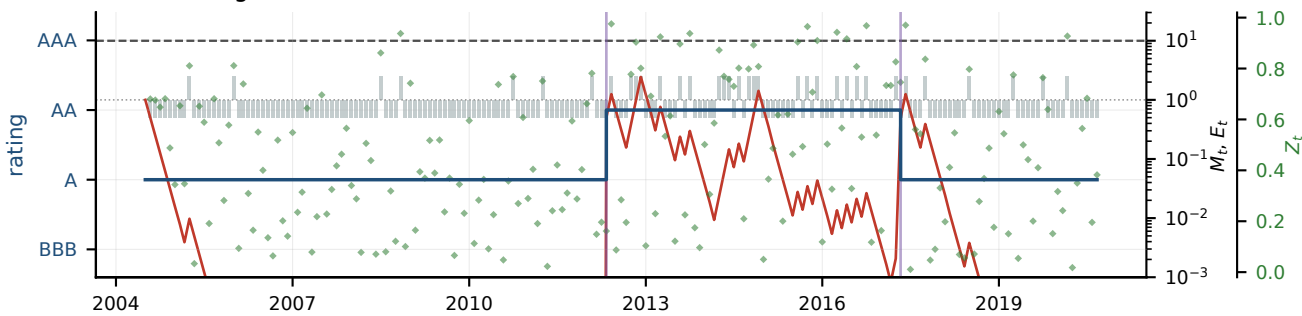
(D) true negative — a quiescent bond, correctly left alone — US25179SAD27
