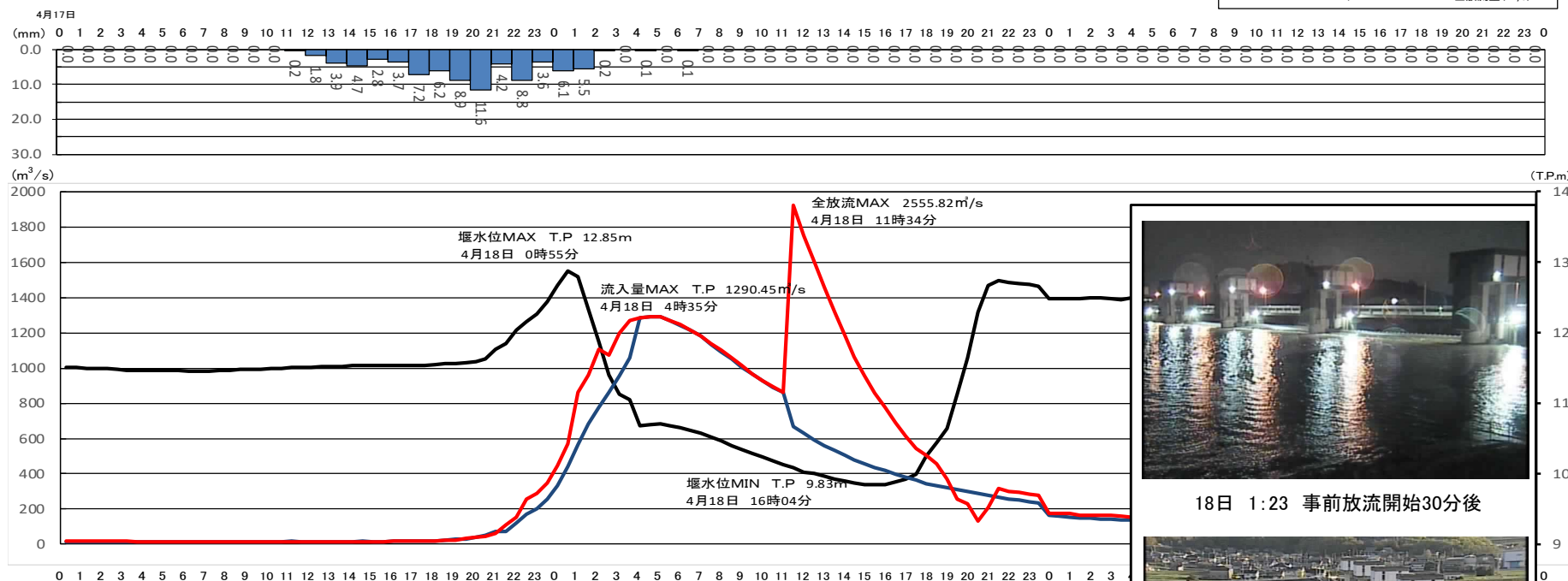
加古川大堰洪水体制時グラフ
