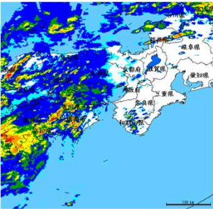
7月4日 12:00 雨量図
