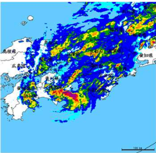
7月4日 15:00 雨量図
