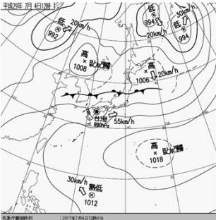
7月4日 12:00 天気図
