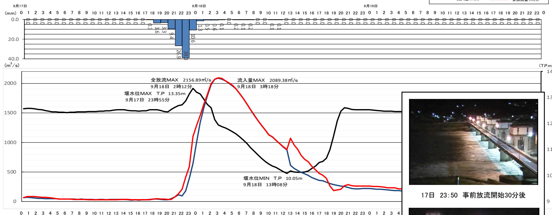
加古川大堰洪水体制時グラフ
