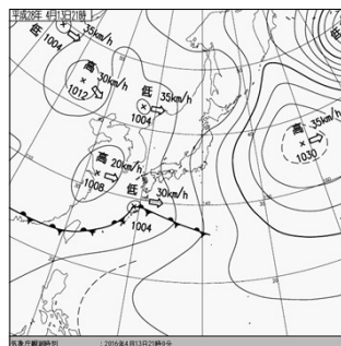
4月13日 21:00 天気図
