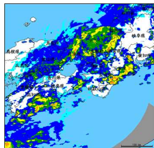
4月13日 21:00 雨量図
