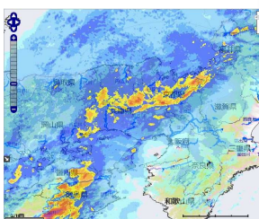
11月2日 12:00 雨量図
