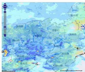
11月2日 12:00 天気図
