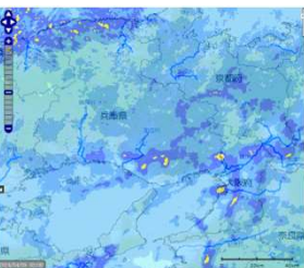
4月9日 3:00 雨量図
