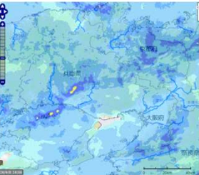
4月9日 0:00 雨量図
