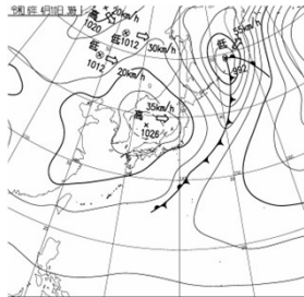
4月9日 3:00 天気図
