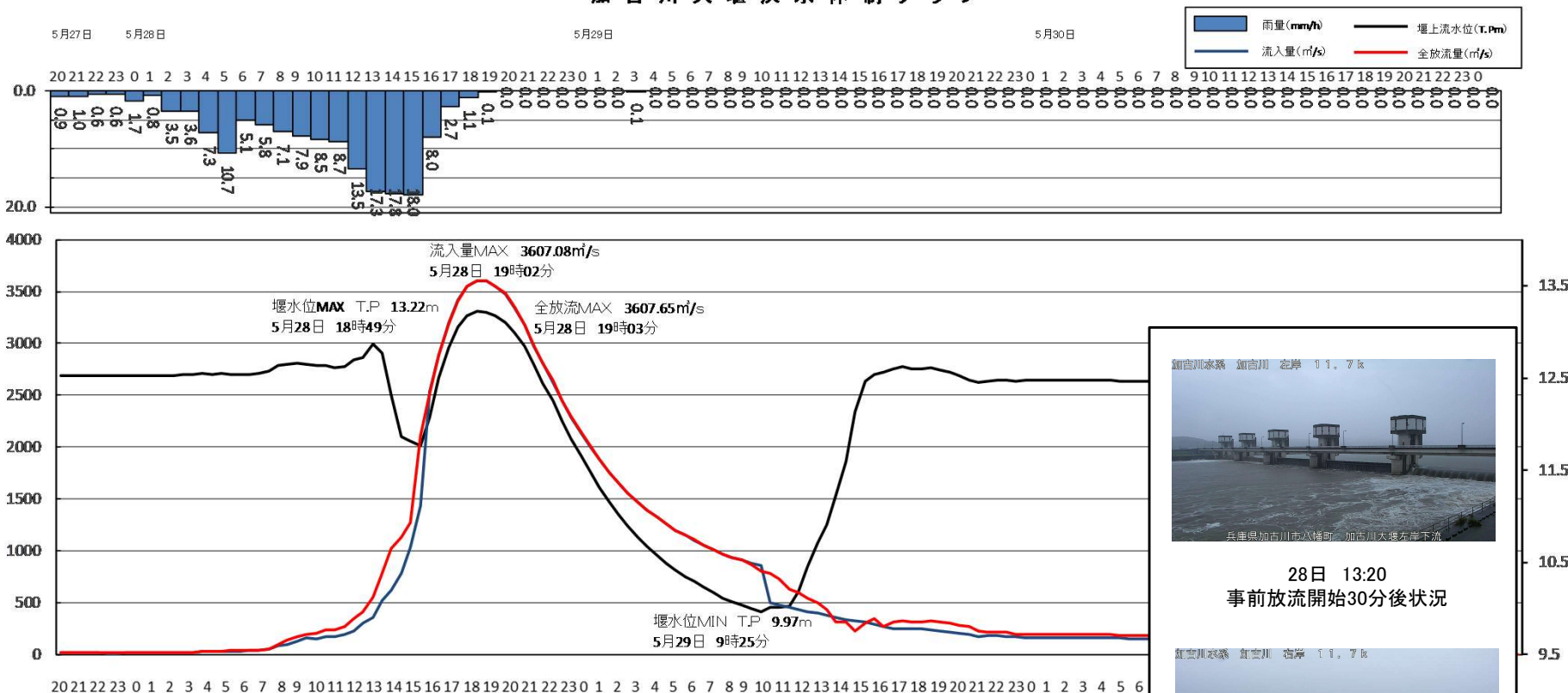
加古川大堰洪水体制グラフ
