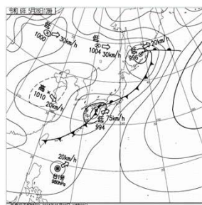
5月28日 12:00 天気図
