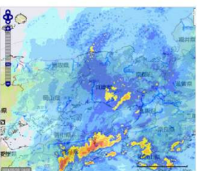
5月28日 14:00 雨量図
