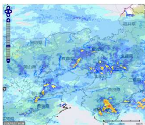
6月28日 4:00 雨量図
