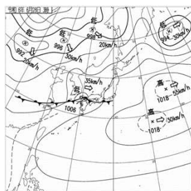
6月28日 3:00 天気図
