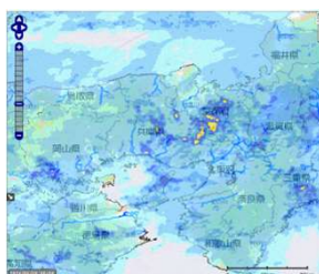
6月28日 5:00 雨量図
