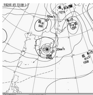
8月7日 12:00 天気図
