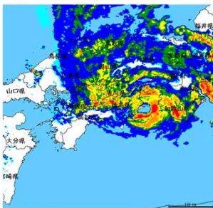
8月7日 13:00 雨量図
