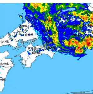
8月7日 16:00 雨量図
