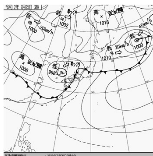
7月25日 3:00 天気図
