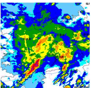
7月25日 3:00 雨量図
