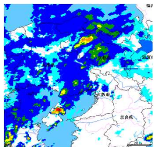
7月24日 14:00 雨量図
