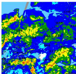
4月29日 12:00 雨量図
