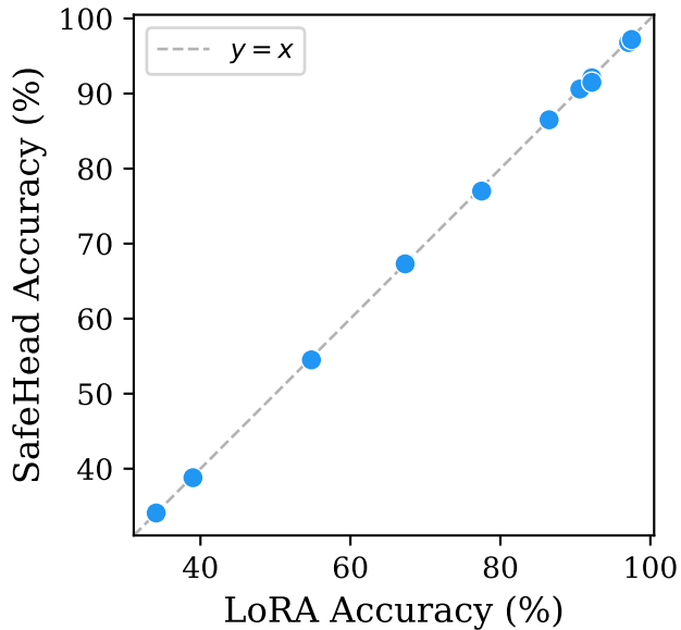
LLaMA-3-8B
