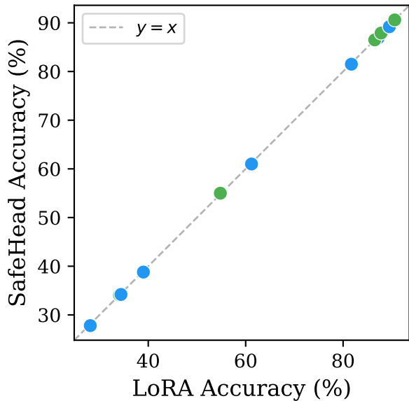
LLaMA-3-8B
