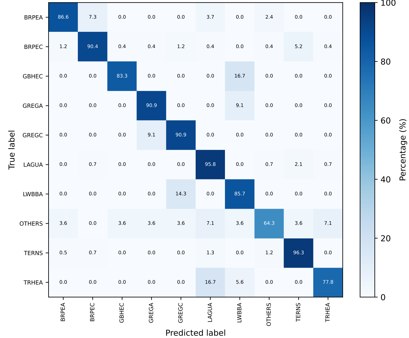
Test
