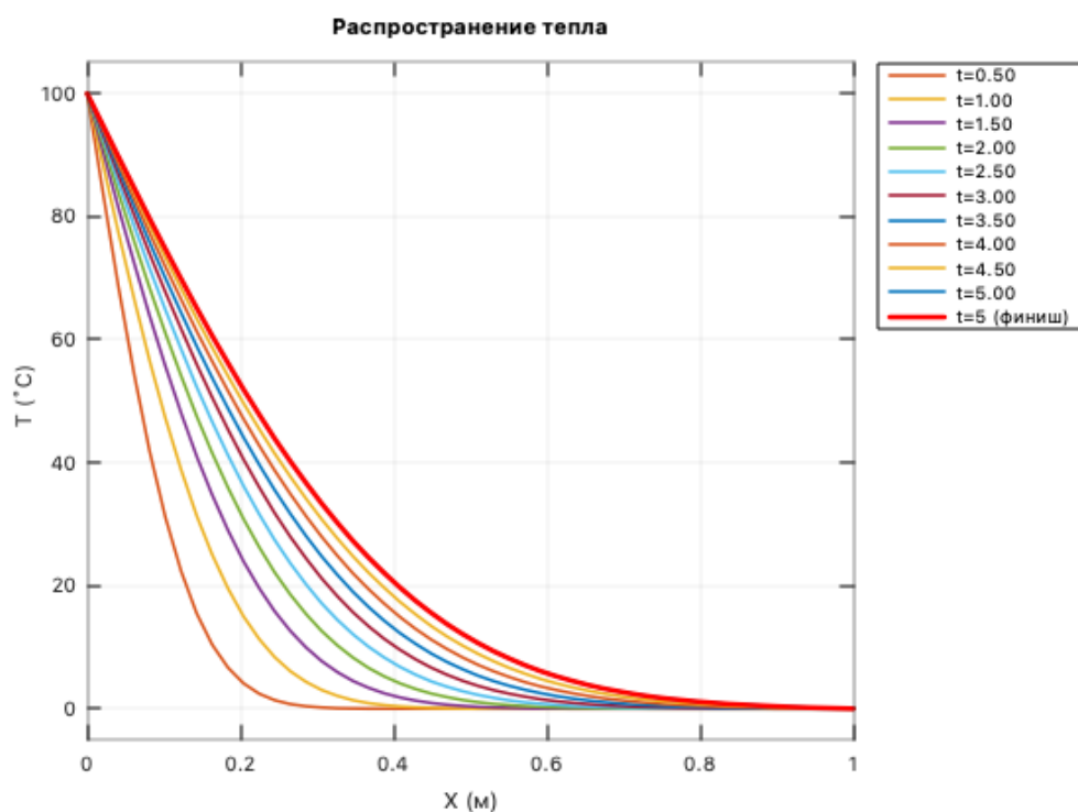
Рис. 1: Распределение температуры вдоль стержня
