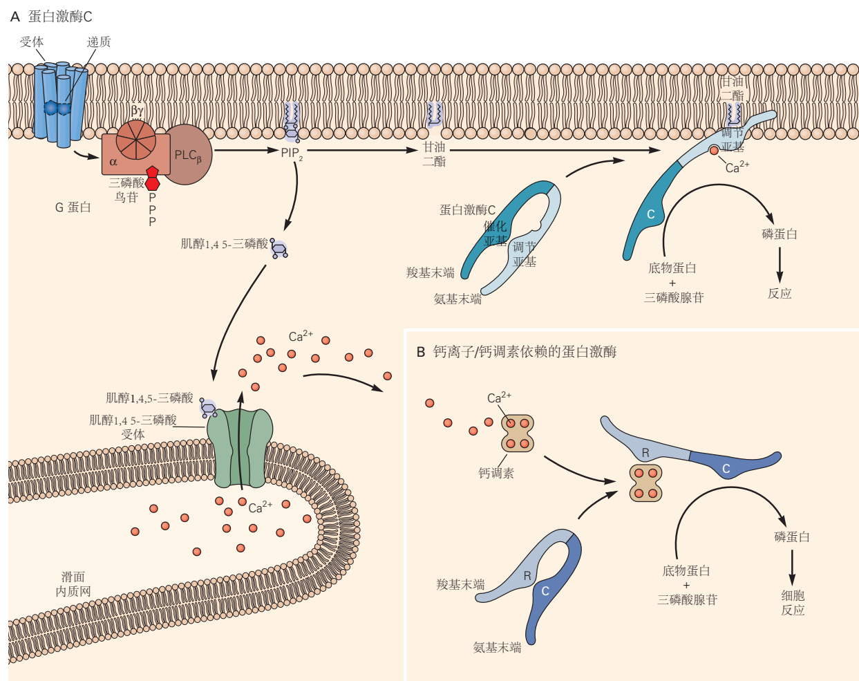
图 14.1.2: 细胞膜中磷脂的水解激活 3 个主要的第二信使级联响应。A. 递质与受体的结合激活了激活磷脂酶 \text{C}_\beta (磷脂酶 \text{C}_\beta ) 的 G 蛋白。这种酶将磷脂酰肌醇-4,5-二磷酸裂解成第二信使肌醇 1,4,5-三磷酸和甘油二酯。肌醇 1,4,5-三磷酸是水溶性的并扩散到细胞质中, 在那里它与光滑内质网上的肌醇 1,4,5-三磷酸受体通道结合, 从而从内部储存中释放 \text{Ca}^{2+} 。甘油二酯保留在膜中, 在那里它募集并激活蛋白激酶 C。膜磷脂也是蛋白激酶 C 激活所必需的辅助因子。蛋白激酶 C 的一些亚型也需要 \text{Ca}^{2+} 才能激活。蛋白激酶 C 由单个蛋白质分子组成, 该分子具有结合甘油二酯的调节结构域和使丝氨酸或苏氨酸残基上的蛋白质磷酸化的催化结构域。在没有甘油二酯的情况下, 调节域会抑制催化域。B. 当 \text{Ca}^{2+} 与钙调蛋白结合时, 钙/钙调蛋白依赖性蛋白激酶被激活, 然后钙/钙调蛋白复合物与激酶的调节域结合。该激酶由许多相似的亚基组成 (此处仅显示其中一个), 每个亚基都具有调节和催化功能。催化结构域磷酸化丝氨酸或苏氨酸残基上的蛋白质。
