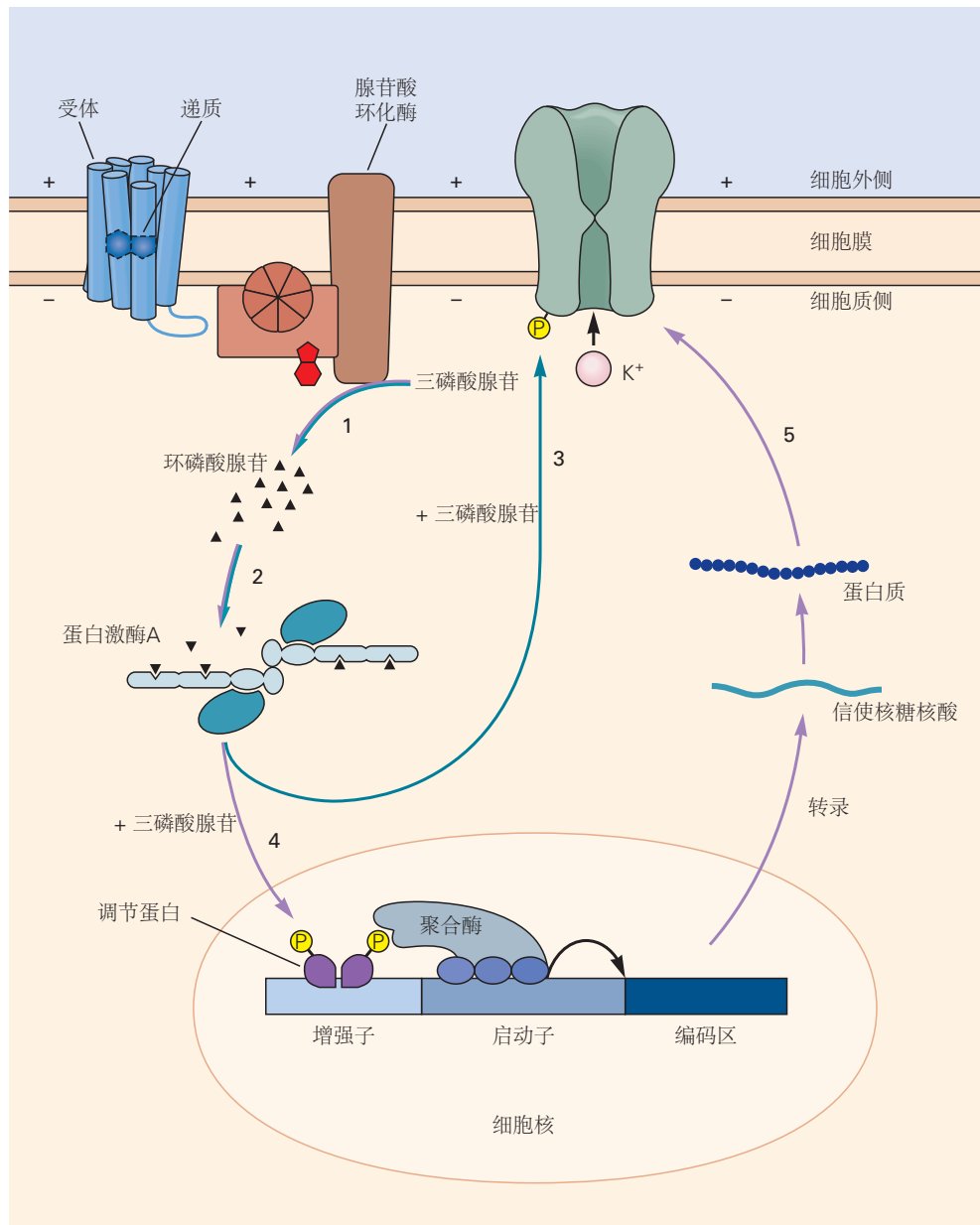
图 14.6.1: 单一神经递质可以对离子通道产生短期或长期的影响。在此示例中，短间接接触递质会激活环磷酸腺苷第二信使系统 (1)，进而激活蛋白激酶 A (2)。激酶磷酸化 K^+ 通道；这会导致持续几分钟的突触电位并改变神经元的兴奋性 (3)。随着受体的持续激活，激酶转移到细胞核，在那里磷酸化一种或多种开启基因表达的转录因子 (4)。作为新蛋白质合成的结果，突触动作被延长，即通道的关闭和神经元兴奋性的变化持续数天或更长时间 (5)。
