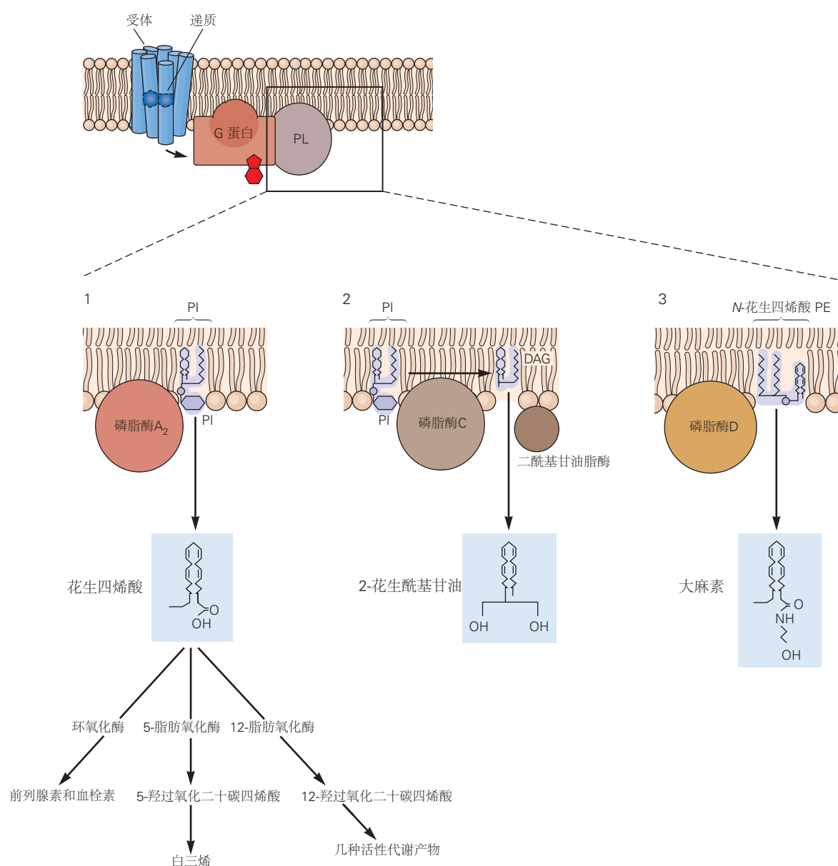
图 14.4.1: 3 种磷脂酶通过水解含有花生四烯酸的磷脂产生不同的第二信使。通路 1. 刺激 G 蛋白偶联受体导致游离 \beta\gamma -亚基复合物激活磷脂酶 A 2 。磷脂酶 A 2 水解细胞质膜中的磷脂酰肌醇，导致释放花生四烯酸，这是一种具有 4 个双键的 20 碳脂肪酸，是许多磷脂的组成部分。一旦释放，花生四烯酸就会通过几种途径代谢，图中显示了其中 3 种。12-脂肪氧化酶通路和 5-脂肪氧化酶通路均产生多种活性代谢物；环氧化酶途径产生前列腺素和血栓素。环氧化酶被吡哌美辛、阿司匹林和其他非甾体类抗炎药抑制。花生四烯酸及其许多代谢物调节某些离子通道的活性。通路 2. 如图 14.1.2 所示，其他 G 蛋白激活磷脂酶 C，后者水解膜中的磷脂酰肌醇生成甘油二酯。第二种酶二酰基甘油酯酶水解甘油二酯，导致产生 2-花生酰基甘油，这是一种从神经元膜释放的内源性大麻素，然后激活其他细胞质膜中的 G 蛋白偶联内源性大麻素受体相邻的神经元。通路 3. 细胞内 Ca 2+ 升高激活磷脂酶 D，后者水解具有异常极性头基的磷脂，其中含有花生四烯酸 (N-花生四烯酸磷脂酰乙醇胺)。该作用会产生第二种内源性大麻素，称为大麻素 (花生四烯基乙醇酰胺)。
