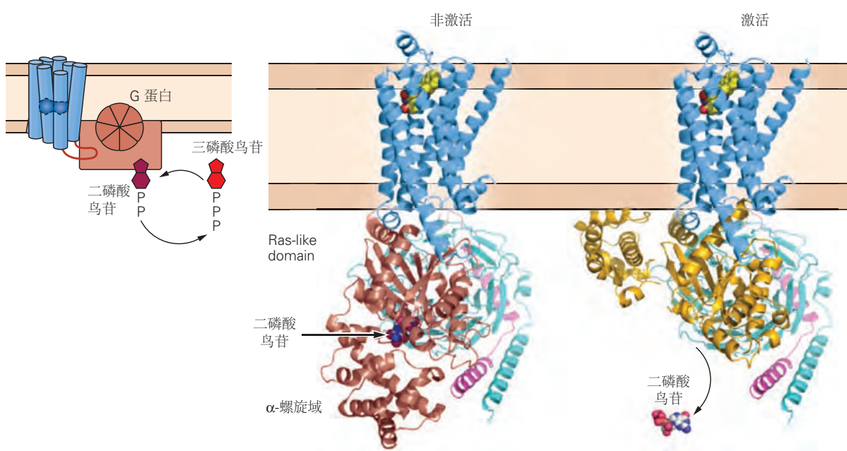
图 14.2.1: G 蛋白偶联受体包含 7 个跨膜结构域。 A. 此处显示的 \beta 2 -肾上腺素能受体代表 G 蛋白偶联受体, 包括 \beta 1 -肾上腺素能和毒蕈碱型乙酰胆碱受体以及视紫红质。它由 1 个具有细胞外氨基末端、细胞内羧基末端和 7 个跨膜 \alpha 螺旋的亚基组成。神经递质的结合位点位于受体中由跨膜螺旋形成的间隙中。氨基酸残基天冬氨酸-113 参与结合。以棕色表示的受体部分与 G_s 蛋白 \alpha 亚基相关。细胞内羧基末端尾部的 2 个丝氨酸残基是特定受体激酶磷酸化的位点, 有助于使受体失活 [82] 。B. 基于 \beta 2 -肾上腺素能受体 (蓝色) 与 G_s 蛋白在非活性二磷酸鸟苷结合状态和活性三磷酸鸟苷结合状态下相互作用的 X 射线晶体结构的模型。高亲和力合成激动剂结合在膜细胞外表面附近的跨膜区域 (空间填充模型)。无活性 G_s 蛋白的 \alpha_s -亚基、 \beta -亚基和 \gamma -亚基分别以棕色、青色和紫色显示。在活性状态下, \alpha_s (金色) 会发生构象变化, 使其能够与腺苷酸环化酶相互作用 [83] 。
