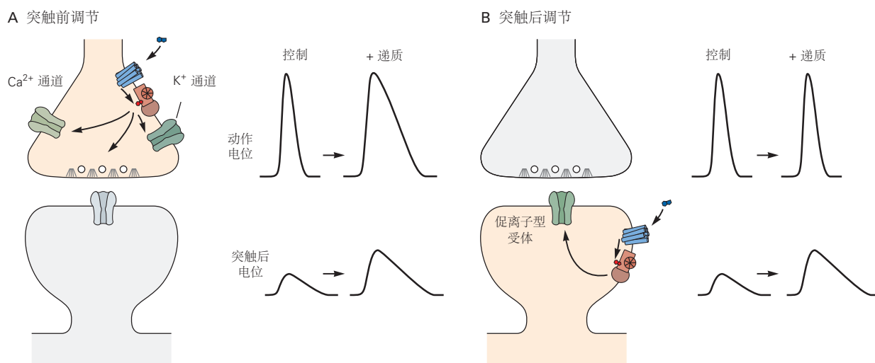
图 14.5.1: 第二信使的调节作用可以通过作用于 2 个突触位点来调节快速突触传递。A. 在突触前末梢，第二信使可以调节递质释放的功效，从而调节由离子型受体介导的快速突触后电位的大小。这可以通过改变突触前 \text{Ca}^{2+} 流入来发生，直接通过调节突触前电压门控 \text{Ca}^{2+} 通道或间接通过调节突触前 \text{K}^{+} 通道，通过控制动作电位持续时间来改变 \text{Ca}^{2+} 流入（如图所示，从而改变 \text{Ca}^{2+} 通道保持开放的时间长度）。一些调制递质直接调节释放机制的功效。B. 在突触后末梢，第二信使可以通过调节离子型受体直接改变突触后电位的幅度。
