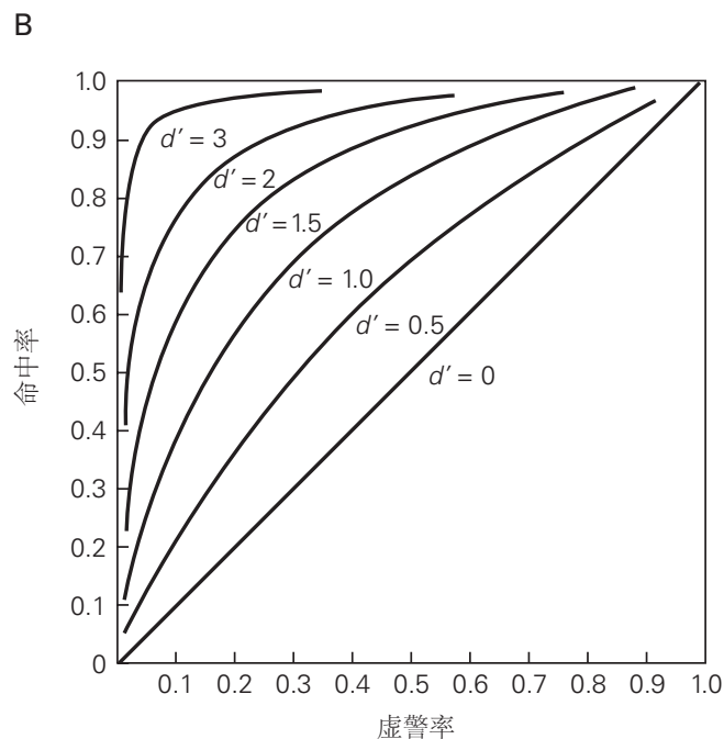
图 17.1.3: 受试者工作特征图显示试验集的结果，每个试验都收集在如图 17.1.2A 所示的矩阵中。垂直轴绘制了命中率或概率作为水平轴上误报率或概率的函数。标记垂直轴真阳性率或灵敏度，以及标记水平轴假阳性率或 (1 - 特异性) 也很常见。随机提供是或否响应的一组试验 (可辨别性 [ d' ] = 0) 绘制为从原点到右上角的直线。这种受试者工作特征的曲线下面积为 0.5。一组完美的试验，其中观察者准确地检测到每个刺激的存在并且不会被任何没有刺激的试验所愚弄 ( d' > 3 )，将沿着左轴急剧上升，并且曲线下面积将为 1.0。曲线下面积越来越多地被引用为单个数字的置信度度量。所示的 (理论) 曲线证明了 d' 的较高值如何导致较大的曲线下面积 [121] 。
