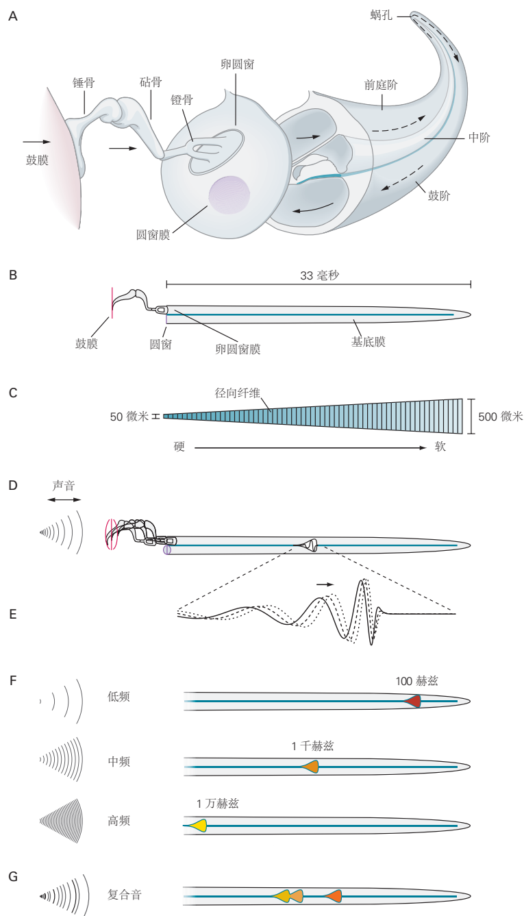
图 26.2.1: 基底膜的运动。 A. 展开的耳蜗，其基部移位以显示其与阶梯的关系，表明刺激能量的流动。声音使鼓膜振动，从而使中耳的 3 个听小骨运动。镫骨的活塞状作用，部分插入弹性椭圆窗的骨头，产生振荡压力差，沿着前庭阶和鼓阶快速传播。低频压力差通过蜗孔分流，2 个管道在这里相通。 B. 如果耳蜗被视为线性结构，只有 2 个由弹性基底膜隔开的充满液体的隔室，则耳蜗的功能特性在概念上得到简化。 C. 此处以表面视图表示的基底膜宽度从基部附近的约 50 微米增加到耳蜗顶端附近的 500 微米。径向胶原纤维从神经到膜的神经外边缘。由于其形态梯度，基底膜的机械性能沿其长度连续变化。 D. 声音的振荡刺激在基底膜上引起行波，此处显示在整个周期内的最大位移范围内。运动幅度在垂直方向上被严重夸大了；可容忍的最大声音仅使基底膜移动 \pm 150 纳米，比例距离小于这些图中代表基底膜的线条宽度的 1/100 。 E. D 中活动区域的扩大表明基底膜响应单频声音刺激的运动。连续曲线描绘了一个瞬间的行波；基底膜偏转的垂直尺度被夸大了大约一百万倍。虚线和虚线曲线描绘了行波在从耳蜗底部（左）向顶点（右）前进时的连续时间。当波接近刺激频率的特征位置时，它会减慢并增加振幅。然后刺激能量被转移到波峰内位置的毛细胞。 F. 每个刺激频率都会在基底膜的特定位置激发最大运动。低频声音会在顶点附近产生基底膜运动，此处的基底膜相对较宽且柔软。中频声音会激发中间的膜。我们能听到的最高频率在其狭窄、僵硬的底部激发基底膜。声频在基底膜上的映射大致呈对数关系。 G. 基底膜对复合的声音进行频谱分析。在此示例中，具有 3 个显著频率的声音（例如元音的 3 个共振峰）会激发 3 个区域的基底膜运动，每个区域代表 1 个特定的频率。相应位置的毛细胞将基底膜振荡转化为受体电位，进而激发支配这些特定区域的神经纤维。
