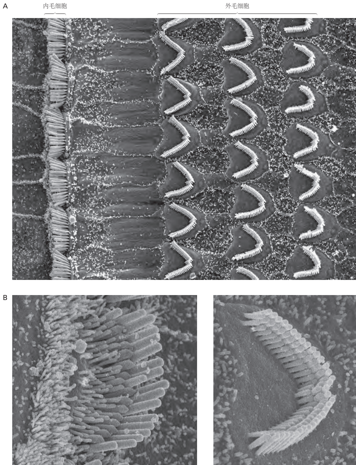
图 26.3.3: 柯蒂氏器中毛细胞的排列。A. 内毛细胞排成一行，每个细胞的静纤毛呈直线排列。相反，外毛细胞呈三排分布，每个细胞的静纤毛呈 V 字型排列。如图 26.3.1 所示，其他几个细胞的顶面可见：从左到右，内螺旋沟细胞、柱状细胞、戴特氏细胞和亨森细胞。B. 更高的放大倍数显示了内毛细胞顶部发状纤维束的线性结构（左）和外毛细胞束的 V 形结构（右），以及静纤毛按高度增加的行排列。
