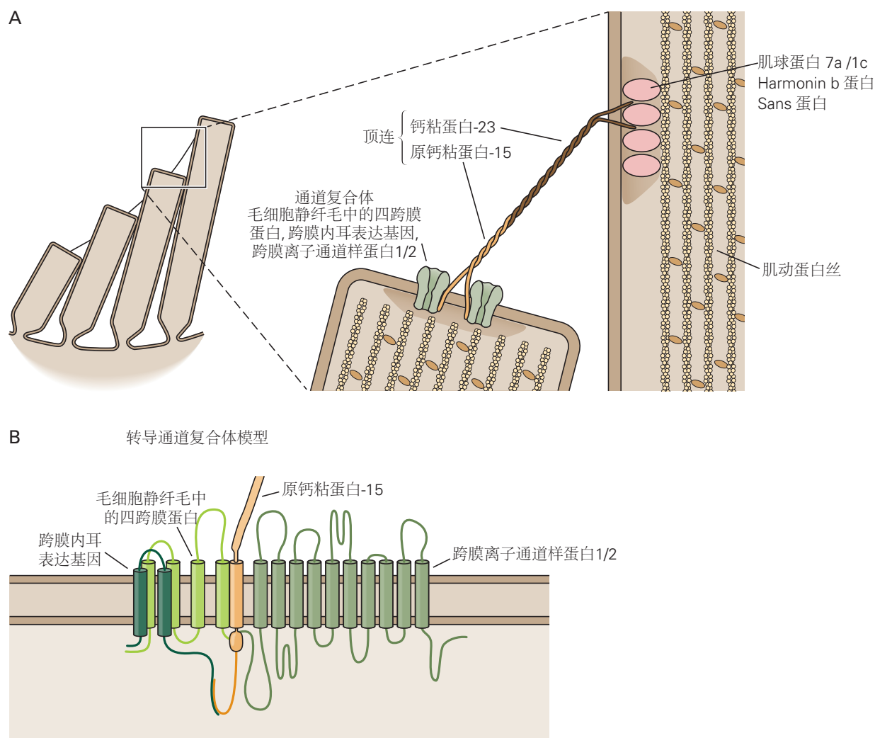
图 26.4.4: 转导机制的分子组成。A. 尖端连接由原钙粘蛋白 15 和钙粘蛋白 23 的异嗜性结合组成。2 个转导通道位于较短的静纤毛尖端连接的下插入点附近。每个通道都是分子复合体的一部分，其中包括蛋白质跨膜离子通道样蛋白 1/2、毛细胞静纤毛中的四跨膜蛋白和跨膜内耳表达基因。在较长静纤毛侧翼的上部插入点，钙粘蛋白 23 与协调蛋白 b 和分子马达肌球蛋白 7a 相互作用，它们都与肌动蛋白结合，从而锚定尖端连接。蛋白质 sans 用作支架蛋白。在前庭毛细胞中，肌球蛋白 1c 可能使尖端连接处于紧张状态，但这种运动蛋白在耳蜗毛细胞中的存在尚不确定。B. 转导通道复合体模型。跨膜离子通道样蛋白 1/2、毛细胞静纤毛中的四跨膜蛋白和跨膜内耳表达基因与原钙粘蛋白 15 相互作用，因此与尖端连接的下端相互作用。跨膜内耳表达基因还与毛细胞静纤毛中的四跨膜蛋白交互。这些蛋白质在转导装置内的详细排列仍然未知。与图中所示不同的是，跨膜离子通道样蛋白 1 被提议组装成二聚体，每个跨膜离子通道样蛋白 1 分子都为阳离子提供渗透通路 [233-234] 。
