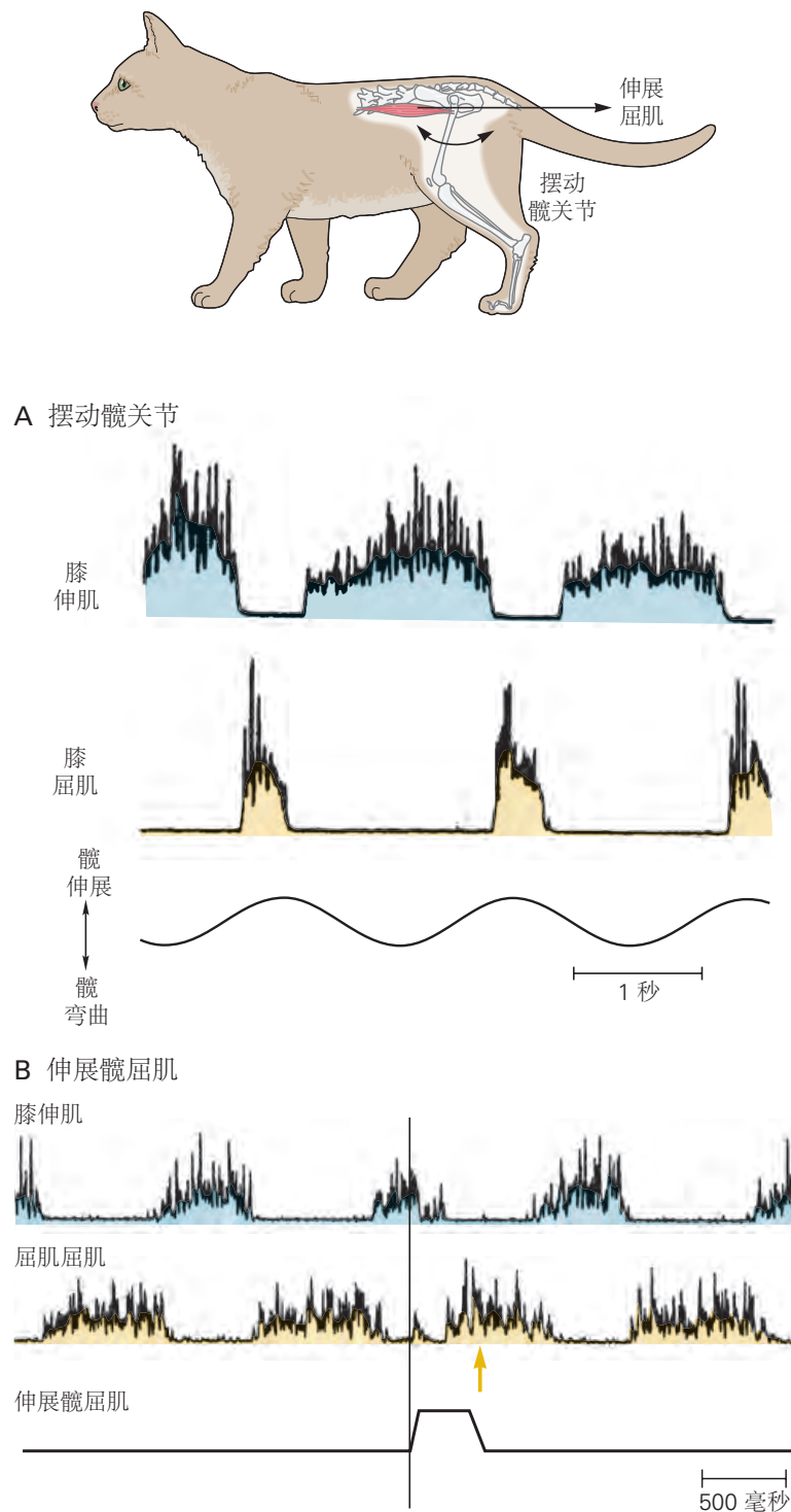
图 33.3.1: 髋关节伸展启动了步行从站立阶段到摆动阶段的转变。A. 在固定的去脑猫中，髋关节周围的被动摆动运动启动并引起膝伸肌和屈肌运动神经元的虚拟移动模式。屈肌肌电图爆发对应于摆动阶段，并在髋关节伸展时产生 [309] 。B. 在行走的去脑猫中，髋屈肌（髂腰肌）的拉伸抑制膝伸肌肌电图活动，使膝屈肌活动更早开始。膝屈肌记录中的箭头表示如果髋屈肌没有被拉伸，肌肉活动何时开始。来自髋屈肌中肌梭的感觉纤维的激活是造成这种效果的原因 [310] 。
