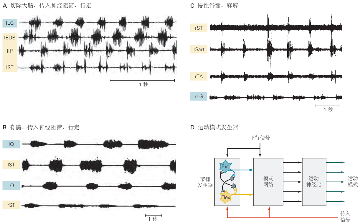
图 33.2.2: 脊髓回路产生节律和模式。A. 即使在通过切断背根去除了脊髓的所有感觉输入之后，在跑步机上行走的去脑猫仍表现出复杂的运动模式，而不仅仅是屈肌和伸肌活动的简单交替 [303] 。B. 左旋多巴和烟肼酰胺的静脉注射在背根被切断的急性脊髓猫中，其产生了组织良好的移动模式 [304] 。C. 慢性脊髓瘫痪猫的虚构移动，展示典型的运动模式在完整猫的半腱肌、胫前肌、外侧胫骨后肌和缝匠肌缝匠肌中 [305] 。D. 基于去脑猫研究的脊髓移动中枢模式发生器的概念模型。中枢模式发生器模型由单独的节律和模式生成层组成。这些层中的每一层都可以通过下行输入和外围传入信息进行修改 [306] 。
