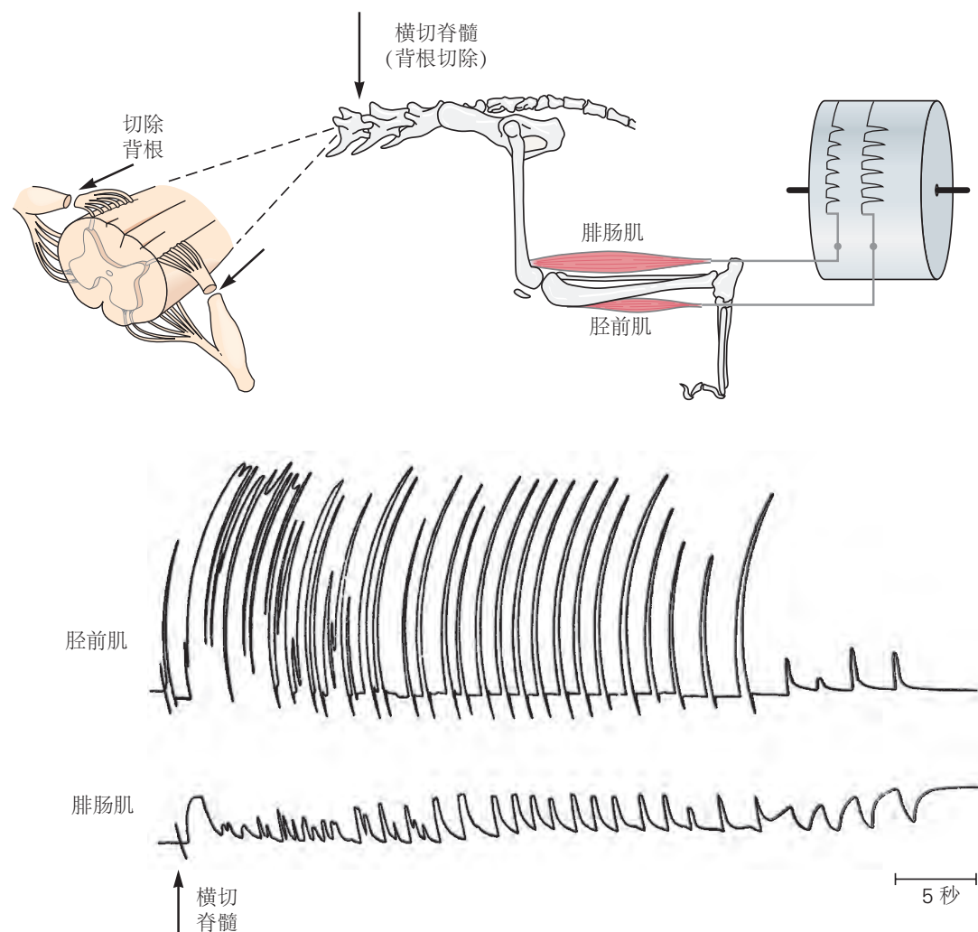
图 33.2.1: 有节律的步进是由脊髓网络产生的。1911 年，托马斯·格拉汉姆·布朗首次证明了内在脊髓网络的存在，他开发了一种实验样品，在该样品中，背根被切断，因此来自肢体的感觉信息无法到达脊髓。下图显示了格拉汉姆·布朗研究中的原始记录。踝关节屈肌（脛骨前肌）和踝关节伸肌（腓肠肌）的节律性交替收缩由孤立的脊髓产生，并在横断后持续一段时间。
