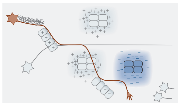
7 旁支
