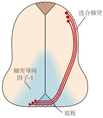
A 野生型
