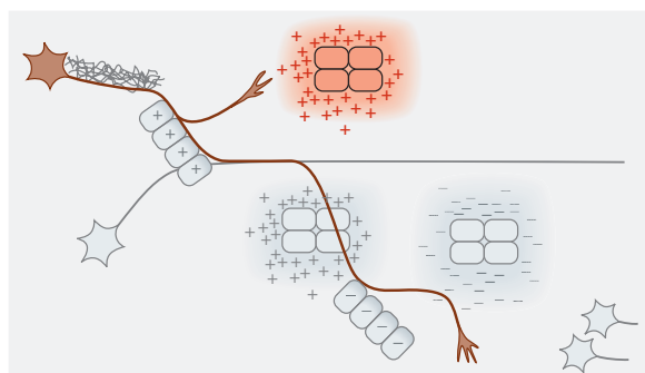
8 终端分支
