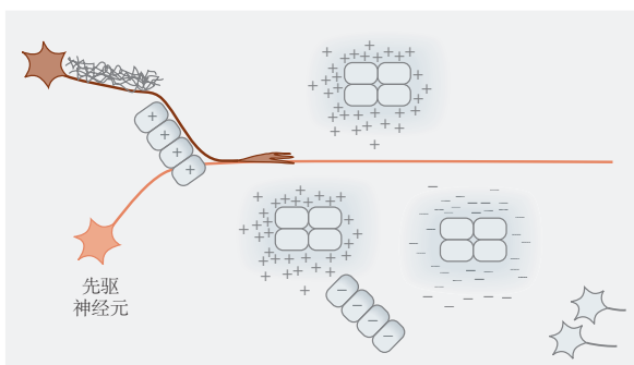
4 化学吸引
