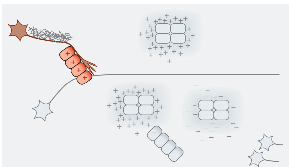
3 束状
