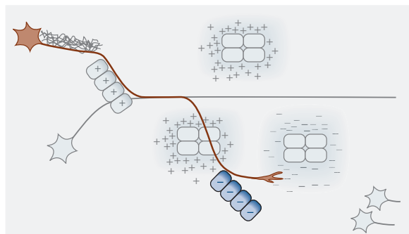
6 化学排斥
