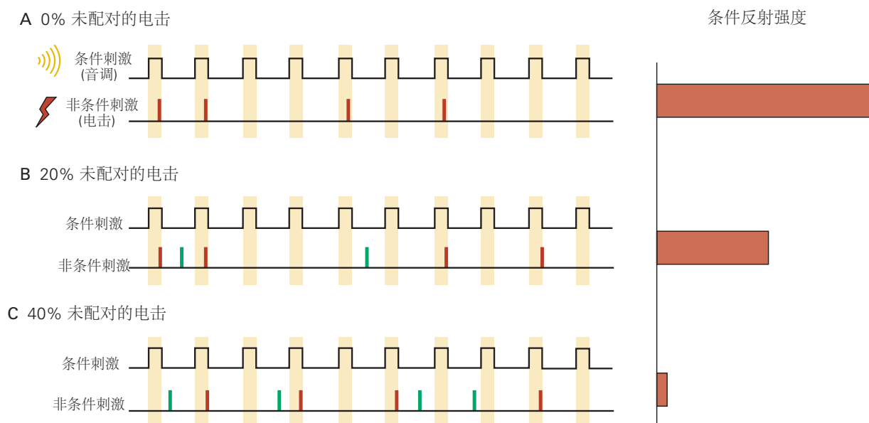
图 52.3.3: 经典条件反射取决于 2 个刺激的相关程度。在这项针对大鼠的实验中, 在 10 项试验中有 4 项 (红色勾号) 将音调 (条件刺激) 与电击 (非条件刺激) 配对。在一些试验块中, 电击是在没有音调 (绿色勾号) 的情况下呈现的。按压杠杆来获得食物的抑制是僵滞的表现, 是一种条件性防御响应。通过确定单独的音调在抑制按下杠杆以获得食物方面的效果来评估调节程度 [496] 。A. 当无条件刺激只接受条件刺激时, 会出现最大条件反射。当没有音调出现电击时几乎和有音调时一样频繁地出现 (40%), 很少或没有条件反射。当 20% 的时间没有音调发生电击时, 就会发生一些条件反射。
