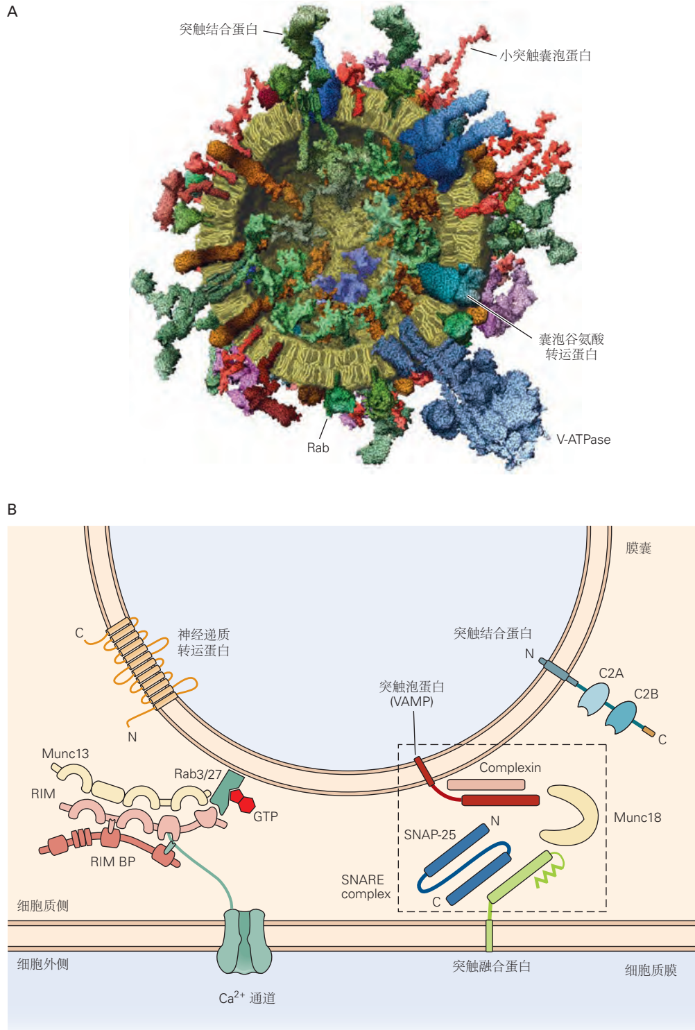
图 15.5.1: 胞吐作用的分子成分。A. 谷氨酸能突触小泡的蛋白质成分描述 (及其近似拷贝数)。蛋白质嵌入突触小泡中, 按比例绘制。成分包括囊泡三磷酸腺苷酶 (每个囊泡 1-2 个)、囊泡谷氨酸转运蛋白 (每个囊泡约 10 个)、小突触囊泡蛋白 (每个囊泡约 70 个)、突触结合蛋白 (每个囊泡约 15 个) 和小 GTPases Rab3 和/或 Rab27。估计值是作为许多囊泡的平均值获得的 [112] 。B. 介导 \text{Ca}^{2+} 触发的囊泡与突触前细胞膜融合的分子机制。这种对停靠突触小泡和突触前活动区的一部分的描述说明了神经递质释放机制的几个关键功能蛋白的相互作用。右图: 虚线框显示核心融合机制, 由可溶性 N-乙基马来酰亚胺敏感因子附着受体蛋白突触泡蛋白/突触小泡缔合性膜蛋白、突触融合蛋白-1 和可溶性 N-乙基马来酰亚胺敏感因子附着受体-25 以及哺乳动物非协调蛋白 18-1 组成。 \text{Ca}^{2+} 传感器突触结合蛋白-1 与 complexin (显示为与可溶性 N-乙基马来酰亚胺敏感因子附着受体复合体结合) 协同作用。左图: 活性区蛋白复合物还包含 Rab 相互作用分子、哺乳动物非协调蛋白 13 和 Rab 相互作用分子结合蛋白以及突触前细胞质膜中的 \text{Ca}^{2+} 通道。Rab 相互作用分子在这个复合物中起着核心作用, 通过结合特定的靶蛋白来协调活性区的多种功能: (1) 囊泡 Rab 蛋白 (Rab3 和 Rab27) 介导囊泡对接; (2) 哺乳动物非协调蛋白 13 激活囊泡启动; (3) \text{Ca}^{2+} 通道, 直接和间接通过 Rab 相互作用分子结合蛋白, 将 \text{Ca}^{2+} 通道束缚在对接囊泡 100 纳米以内。活性区蛋白复合物将关键元素放入附近, 使囊泡能够快速停靠、引发和融合, 以响应动作电位, 触发的 \text{Ca}^{2+} 进入停靠囊泡附近 [113] 。
