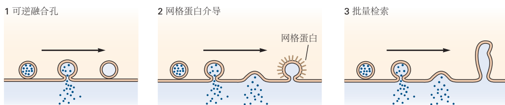
图 15.4.5: 突触小泡周期。A. 突触小泡通过主动运输充满神经递质（第 1 步）并加入可能代表储备池的小泡簇（第 2 步）。填充的囊泡停靠在活性区（第 3 步），在那里它们经历三磷酸腺苷依赖性启动响应（第 4 步），使它们能够进行 \text{Ca}^{2+} 触发的融合（第 5 步）。释放内容物后，突触小泡通过几种通路之一循环（参见 B 部分）。在一种常见的通路中，囊泡膜通过网格蛋白介导的内吞作用（步骤 6）回收并直接回收（步骤 7）或通过核内体（步骤 8）回收。B. 递质放电后囊泡的恢复被认为是通过 3 种机制发生的，每种机制都有不同的动力学。1. 可逆融合孔是再利用囊泡的最快速机制。囊泡膜不与细胞质膜完全融合，递质通过融合孔释放。囊泡回收只需要关闭融合孔，因此可以在数十到数百毫秒内迅速发生。该通路可能在较低至正常的释放速率下占主导地位。用过的囊泡可能会留在膜上（亲吻和停留）或从膜重新定位到囊泡储备池（亲吻和奔跑）。2. 在经典通路中，多余的膜通过网格蛋白包被的小坑通过内吞作用回收。除了活动区外，这些凹坑遍布整个轴突末梢。该通路在正常到高释放率下可能很重要。3. 在大量回收通路中，多余的膜通过未包被的凹坑出芽重新进入末梢。这些未涂层的池主要在活动区形成。该通路可能仅在高释放率之后使用，而不是在突触的正常功能期间使用 [111] 。
