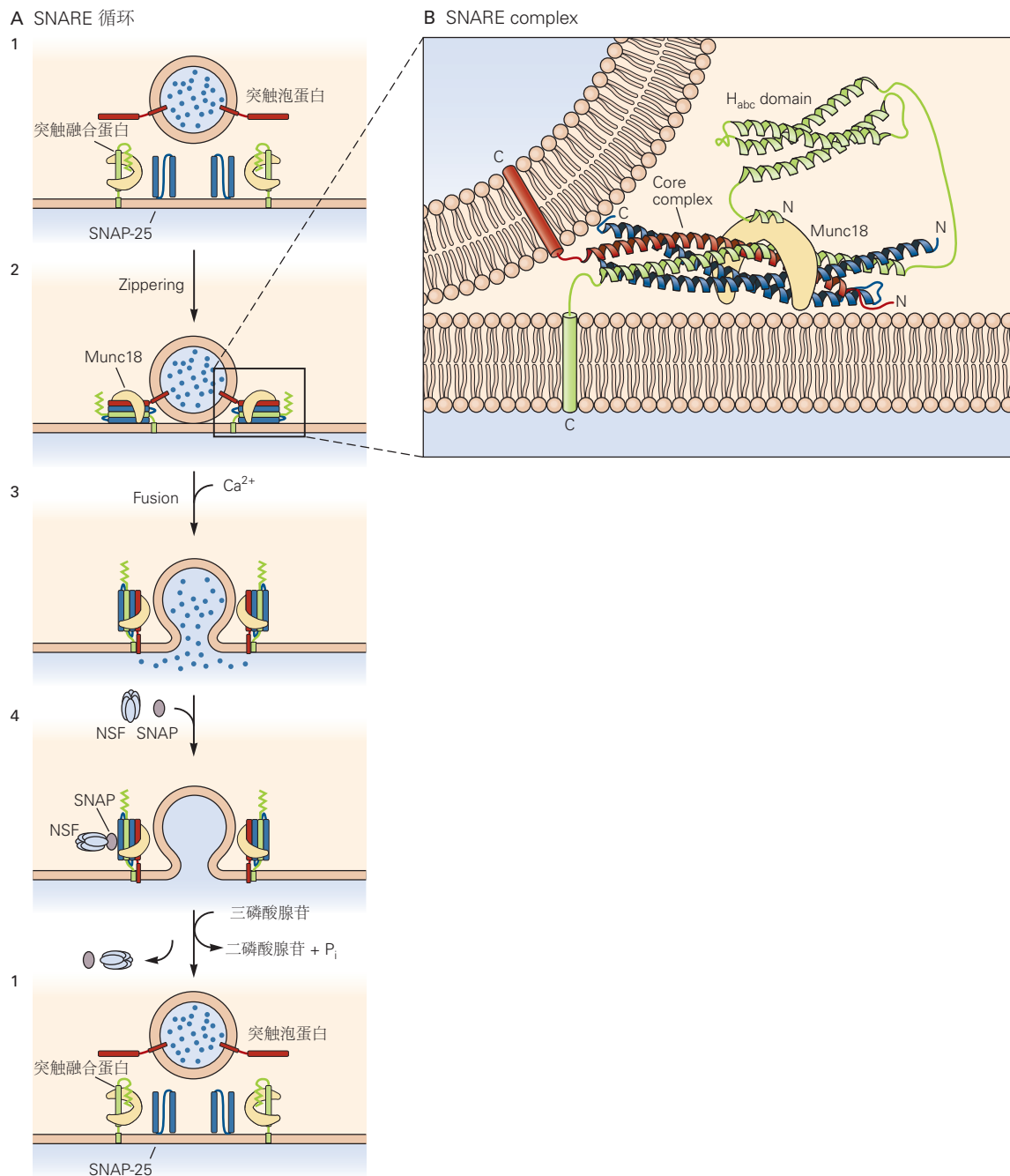
图 15.5.2: 可溶性 N-乙基马来酰亚胺敏感因子附着受体复合体的形成和解离驱动突触小泡和细胞质膜的融合 [114] 。A. 可溶性 N-乙基马来酰亚胺敏感因子附着受体循环。1. 突触泡蛋白与 2 种细胞质膜蛋白相互作用，即跨膜蛋白突触融合蛋白和外周膜蛋白可溶性 N-乙基马来酰亚胺敏感因子附着受体-25。2. 这 3 种蛋白质形成紧密的复合物，使囊泡和突触前膜紧密并列。哺乳动物非协调蛋白 18 与可溶性 N-乙基马来酰亚胺敏感因子附着受体复合体结合。3. \text{Ca}^{2+} 流入引发囊泡和细胞质膜的快速融合；可溶性 N-乙基马来酰亚胺敏感因子附着受体复合体现在位于细胞质膜中。4. 2 种蛋白质 N-乙基顺丁烯二酰亚胺敏感性的融合蛋白和可溶性 N-乙基马来酰亚胺敏感因子附着受体（与可溶性 N-乙基马来酰亚胺敏感因子附着受体-25 无关）与可溶性 N-乙基马来酰亚胺敏感因子附着受体复合体结合并导致它在三磷酸腺苷依赖性响应中解离。B. 可溶性 N-乙基马来酰亚胺敏感因子附着受体复合体由一束 4 个 \alpha -螺旋组成，一个来自突触泡蛋白和突触融合蛋白，2 个来自可溶性 N-乙基马来酰亚胺敏感因子附着受体-25。这里显示的结构是融合前的停靠囊泡（跨膜结构域的实际结构尚未确定，但出于说明目的，此处将结构域与囊泡和细胞质膜一起绘制）。
