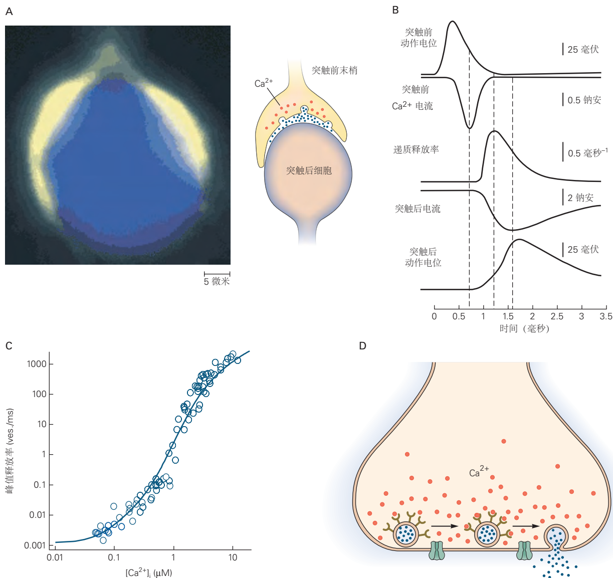
图 15.2.3: 已经测量了突触前 \text{Ca}^{2+} 与中央突触中递质释放之间的精确关系 [97-98] 。A. 哺乳动物中花萼突触的大突触前末梢，脑干吞没突触后细胞体。左侧的荧光图像显示了一个充满 \text{Ca}^{2+} 敏感染料的花萼。B. 几个突触事件的时间进程。虚线表示 \text{Ca}^{2+} 电流、递质释放和突触后电流的峰值响应时间。C. 递质释放高度依赖于突触前末梢的 \text{Ca}^{2+} 浓度。花萼装有笼状 \text{Ca}^{2+} 化合物，该化合物可响应紫外线闪光释放其结合的 \text{Ca}^{2+} ，并装有 \text{Ca}^{2+} 敏感染料，可测量细胞内 \text{Ca}^{2+} 浓度。通过控制光的强度，可以调节突触前末梢 \text{Ca}^{2+} 的增加。该图以对数标度显示囊泡释放速率与细胞内 \text{Ca}^{2+} 浓度之间的关系。蓝线描绘了一个模型的数据拟合，该模型假定释放是由结合 5 个 \text{Ca}^{2+} 的主要 \text{Ca}^{2+} 传感器触发的，导致 \text{Ca}^{2+} 协同性为 5。由于 \text{Ca}^{2+} 和释放之间的非线性关系，浓度超过 1 微摩尔时 \text{Ca}^{2+} 的小增量会导致释放大量增加。D. 从囊泡中释放递质需要 5 个 \text{Ca}^{2+} 与 \text{Ca}^{2+} 敏感突触囊泡蛋白结合。在图中， \text{Ca}^{2+} 与单个囊泡上存在的 5 个受体结合；实际上，每个受体分子结合多个 \text{Ca}^{2+} 。
