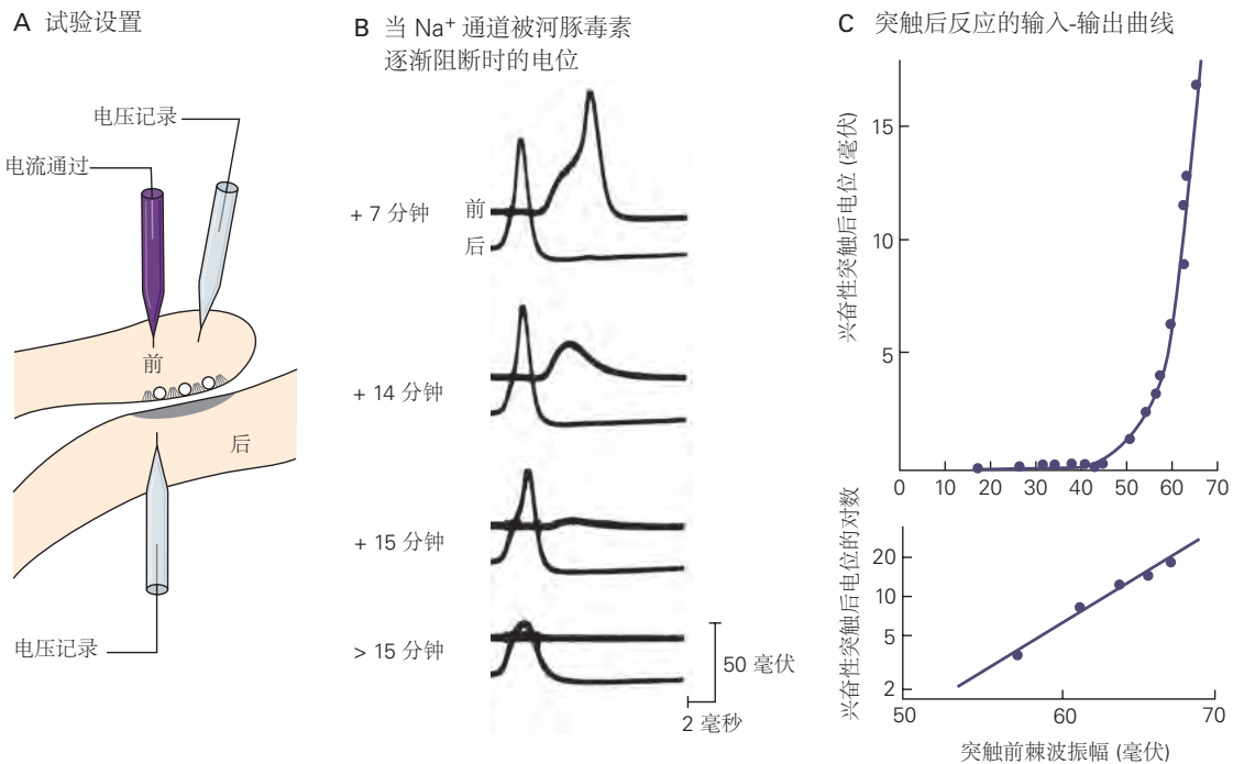
图 15.1.1: 递质释放由突触前膜电位的变化触发 [93] 。A. 电压记录电极插入鱿鱼星状神经节中巨型突触的突触前纤维和突触后纤维。电流通过电极也插入突触前引发了突触前动作电位。B. 将河豚毒素添加到浸泡细胞的溶液中，以阻断作为动作电位基础的电压门控 \text{Na}^+ 通道。随着越来越多的 \text{Na}^+ 通道被阻断，突触前动作电位和兴奋性突触后电位的振幅逐渐降低。7 分钟后，突触前动作电位仍可产生超阈值的兴奋性突触后电位，触发突触后细胞的动作电位。大约 14 到 15 分钟后，突触前脉冲逐渐变小并产生较小的突触后去极化。当突触前峰值降低到 40 毫伏或更低时，它无法产生兴奋性突触后电位。因此，突触前去极化的大小（此处由动作电位提供）控制递质释放的幅度。C. 兴奋性突触后电位振幅对突触前动作电位振幅的依赖性递质释放输入-输出曲线的基础。这种关系是通过在河豚毒素阻断突触前 \text{Na}^+ 通道开始期间刺激突触前神经获得的，此时突触前动作电位和突触后去极化的幅度逐渐降低。上图表明产生突触后电位需要 40 毫伏的突触前动作电位。超过这个阈值，兴奋性突触后电位的振幅会急剧增加，以响应突触前电位振幅的小幅增加。突触前脉冲和兴奋性突触后电位之间的关系是对数关系，如下图所示。突触前脉冲增加 13.5 毫伏会使兴奋性突触后电位增加 10 倍。
