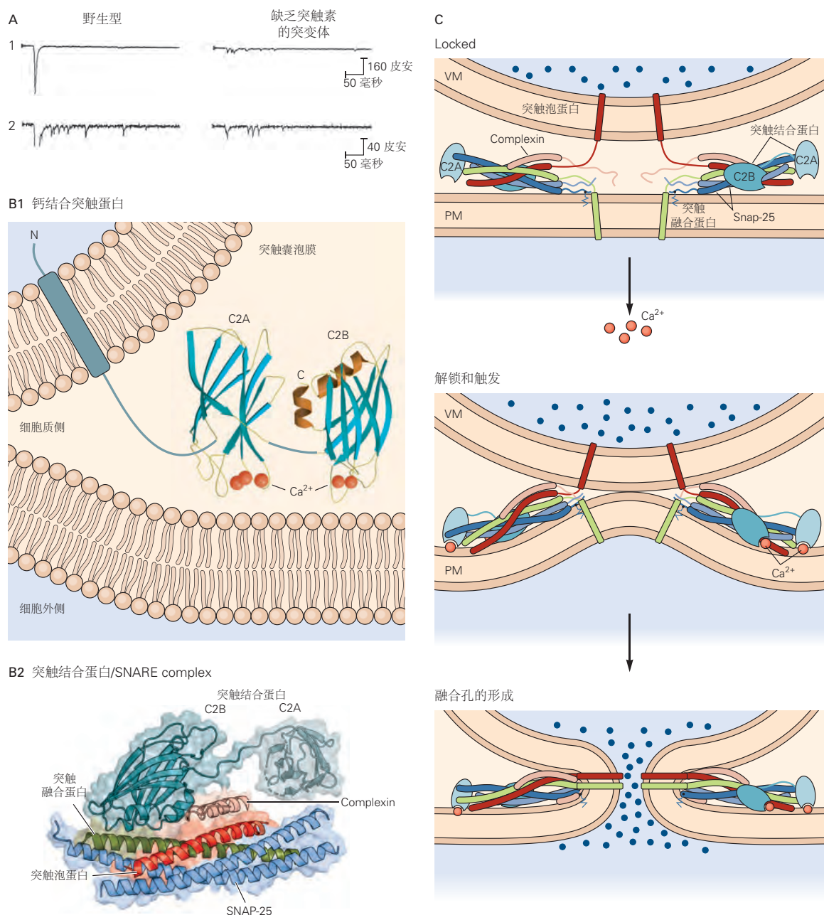
图 15.5.3: 突触结合蛋白通过形成有利于囊泡融合的蛋白质复合物来介导 Ca^{2+} 依赖性递质释放。A. 缺乏突触结合蛋白-1 的突变小鼠不存在快速 Ca^{2+} 触发的递质释放。记录显示兴奋性突触后电流通过刺激来自野生型小鼠和突变小鼠的培养的海马体神经元在体外诱发，其中突触结合蛋白-1 已通过同源重组 (1) 被删除。来自野生型小鼠的神经元显示出由突触前动作电位诱发的大而快速的兴奋性突触后电流，反映了突触传递受大量突触小泡快速同步释放递质支配的事实。在底部轨迹 (2) 中，突触电流以高度扩展的比例显示，可以看到同步释放的快速阶段之后是一个小的、延长的递质异步释放阶段。在这个缓慢的阶段，个体量子响应的频率会持续增加。在突变小鼠的神经元中，突触前动作电位仅触发缓慢的异步释放阶段；快速同步阶段已被废除 [115] 。B. X 射线晶体结构突触结合蛋白。B1. 带状图显示 C2A 结构域结合 3 个 Ca^{2+} ，C2B 结构域结合 2 个 Ca^{2+} 。蓝色箭头表示 \beta 链。在 C2B 结构域的 C 末梢有 2 个短的 \alpha -螺旋 (橙色)。突触结合蛋白其他区域的结构尚未确定，在此绘制以供说明之用。膜和结构按比例绘制 [116] 。B2. 与可溶性 N-乙基马来酰亚胺敏感因子附着受体复合物 (突触泡蛋白、突触融合蛋白和可溶性 N-乙基马来酰亚胺敏感因子附着受体-25) 和 complexin 结合的突触结合蛋白 (浅蓝色) 的 X 射线晶体结构。未显示突触结合蛋白的跨膜结构域 [117] 。C. 突触结合蛋白-复合蛋白-可溶性 N-乙基马来酰亚胺敏感因子附着受体复合物的拉链介导囊泡融合。顶部，在没有 Ca^{2+} 的情况下，可溶性 N-乙基马来酰亚胺敏感因子附着受体复合体和复合体的 \alpha -螺旋与结合的突触结合蛋白仅部分拉开。中间， Ca^{2+} 与突触结合蛋白的 C2A 和 C2B 结构域的结合使它们能够与细胞质膜相互作用，施加力使囊泡和细胞质膜靠得更近。底部，突触结合蛋白介导的接近和复合物-可溶性 N-乙基马来酰亚胺敏感因子附着受体-突触结合蛋白复合物的最终拉链触发膜融合 [117] 。
