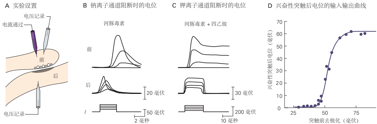
图 15.1.2: 递质释放不是由突触前电压门控 \text{Na}^+ 或 \text{K}^+ 通道的打开直接触发的 [93] 。A. 电压记录电极插入鱿鱼星状神经节中巨型突触的突触前纤维和突触后纤维。电流通过电极也插入突触前细胞。B. 通过微电极直接注入电流使突触前末梢去极化，即使通过向细胞沐浴液中添加河豚毒素完全阻断电压门控 \text{Na}^+ 通道后，也可以触发递质释放。3 组迹线表示（从下到上）注入突触前末梢的去极化电流脉冲（I）、突触前末梢产生的电位（Pre）以及递质释放到突触后细胞上产生的兴奋性突触后电位。突触前细胞中逐渐增强的电流脉冲会相应地产生更大的突触前末梢去极化。突触前去极化越大，兴奋性突触后电位越大。突触前去极化不会在整个去极化电流脉冲的整个持续时间内保持，因为电压门控 \text{K}^+ 通道的延迟激活会导致复极化。C. 即使在电压门控 \text{Na}^+ 通道已被河豚毒素阻断并且电压门控 \text{K}^+ 通道已被四乙铵阻断后，也会发生递质释放。在这个实验中，四乙铵被注入突触前末梢。这 3 组迹线代表与 B 部分相同的测量值。由于突触前 \text{K}^+ 通道被阻断，因此在整个电流脉冲中保持突触前去极化。大量持续的突触前去极化产生大量持续的兴奋性突触后电位。D. 阻断 \text{Na}^+ 和 \text{K}^+ 通道可以准确控制突触前电压并确定完整的输入-输出曲线。超过某个阈值（相对于静息电位为 40 毫伏正值），从兴奋性突触后电位的大小测量，突触前去极化和递质释放之间存在陡峭的关系。大于一定水平的去极化不会导致递质的任何额外释放。最初的突触前静息膜电位约为 -70 毫伏。
