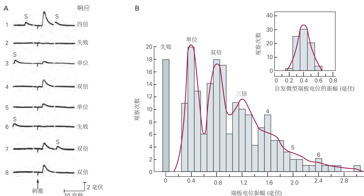
图 15.3.1: 神经递质以固定增量释放。递质的每个增量或量程都会产生一个固定振幅的单位终板电位。因此，神经刺激引起的响应幅度等于单位终板电位的幅度乘以释放的递质的量子数。A. 终板肌纤维的细胞内记录显示：当对运动神经施加 8 个相同大小的连续刺激时，突触后电位发生变化。为了减少递质释放并保持终板电位较小，将组织浸泡在缺乏 \text{Ca}^{2+} （和富含镁）的溶液中。对神经刺激的突触后响应各不相同。8 个突触前刺激中的 2 个不引发兴奋性突触后电位（失败），2 个产生单位电位，其他产生的兴奋性突触后电位大约是单位电位振幅的 2 到 4 倍。请注意，在迹线中以随机间隔出现的自发微型终板电位（S）与单位电位的大小相同 [99] 。B. 在记录了许多终板电位后，在此处显示的直方图中，将具有给定振幅的响应数量绘制为该振幅的函数。响应的分布分为多个峰值。第一个峰值为 0 毫伏，表示失败。第一个响应峰值为 0.4 毫伏，代表单位电位，即最小的引发响应。单位响应与自发的微型终板电位（插图）具有相同的幅度，表明单位响应是由单个递质量子的释放引起的。直方图中的其他峰是单位电位振幅的整数倍；也就是说，响应由 2 个、3 个、4 个或更多的量子事件组成。每个峰值下的响应数除以整个直方图中的事件总数是单个突触前动作电位触发释放构成峰值的量子数概率。例如，如果在记录的总共 100 个事件中，峰值中有 30 个事件对应于 2 个量子的释放，则突触前动作电位恰好释放 2 个量子的概率为 30/100 或 0.3。该概率服从泊松分布（红色曲线）。这个理论分布由几个高斯函数的总和组成。单位峰值的分布（高斯函数的标准偏差）反映了一个事实，即量子中的递质数量，以及量子突触后响应的振幅，围绕平均值随机变化。连续的高斯峰逐渐变宽，因为与每个量子事件相关的可变性（或方差）随着每个事件的量子数量线性增加。自发微型电位（插图）的振幅分布由高斯曲线拟合，其宽度与单位突触响应的高斯曲线宽度相同 [100] 。
