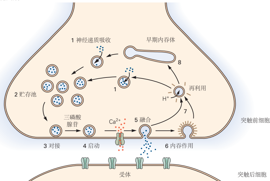
A 突触囊泡周期
