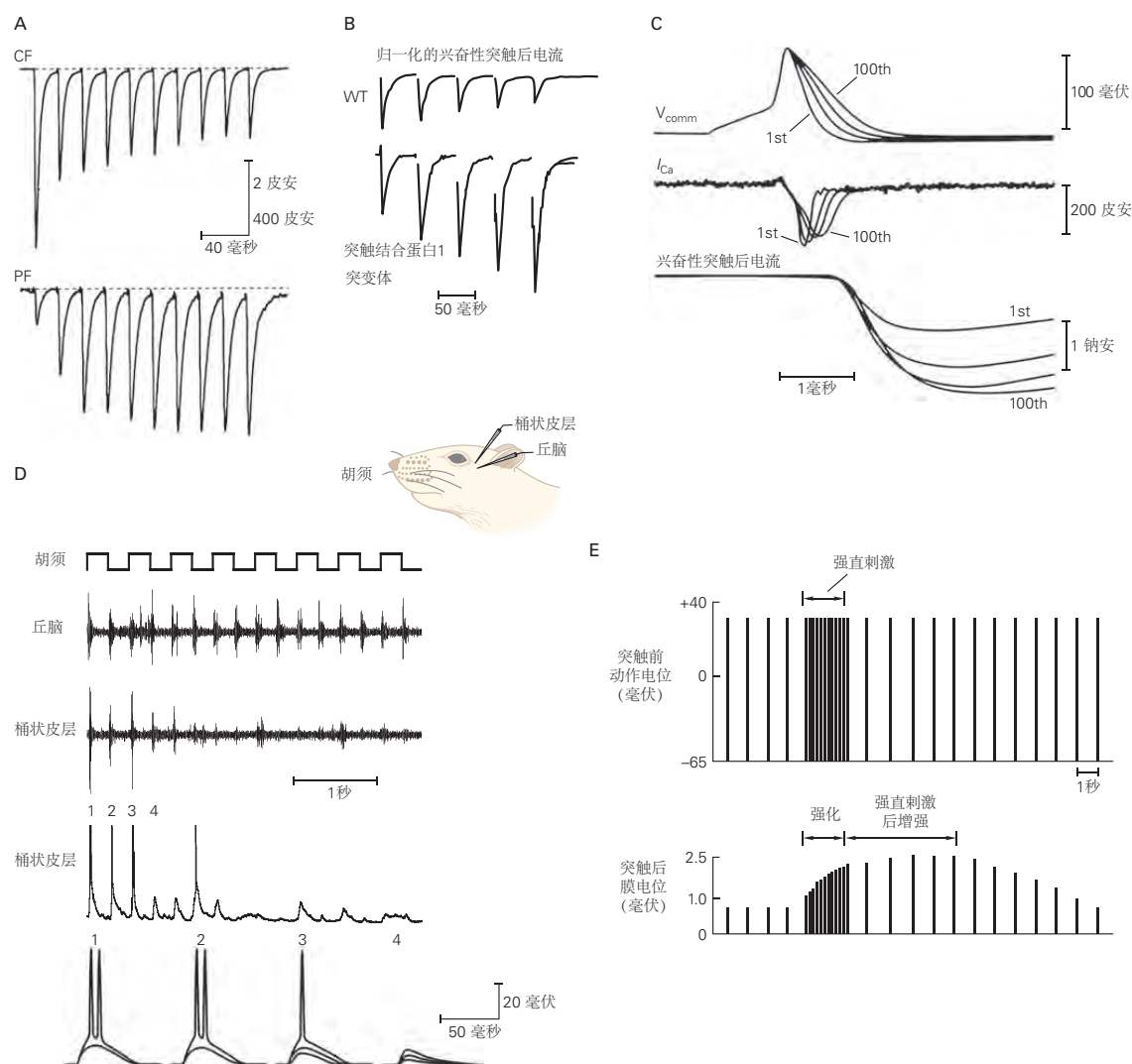
图 15.4.1: 中枢神经系统短期可塑性的多样性。A. 兴奋性突触后电流是在电压钳下从小脑浦肯野神经元记录的，以响应对浦肯野细胞的攀缘纤维或平行纤维输入的重复刺激。在这 2 种情况下，兴奋性突触后电流都被记录下来，而传入神经在 50 赫兹下被刺激 10 次。请注意，攀缘纤维兴奋性突触后电流抑制而平行纤维兴奋性突触后电流在重复刺激期间促进 [102] 。B. 兴奋性突触后电流在 20 赫兹的刺激过程中从培养的海马体神经元中记录下来。通过将每个响应除以每个单独序列中第一个兴奋性突触后电流的峰值振幅，将兴奋性突触后电流大小归一化。兴奋性突触后电流抑制从野生型小鼠培养的神经元，而兴奋性突触后电流促进来自携带突变形式的突触结合蛋白-1 的小鼠的神经元，该突触结合蛋白-1 降低其 \text{Ca}^{2+} 结合亲和力（突触结合蛋白 1 突变体，R233Q） [103] 。C. 在 2 秒长的 50 赫兹刺激序列中，齿状回颗粒神经元突触前末梢记录的动作电位逐渐变宽。这导致从颗粒神经元到它们的阿蒙角 3 突触后目标的突触传递增强。显示第 1、25、50 和 100 个动作电位。然后将这些动作电位波形用作命令波形 ( V_{\text{comm}} ，顶部) 以电压钳制突触前神经末梢（“动作电位钳”），引发末梢（中间）和突触后阿蒙角 3 神经元中的兴奋性突触后电流（底部）。随着动作电位波形持续时间的增加， I_{\text{Ca}} 的持续时间增加，从而增加了兴奋性突触后电流的振幅 [104] 。D. 在对初级胡须进行一系列 4 赫兹机械刺激（顶部迹线）期间，同时对丘脑和桶状皮层的动作电位进行细胞外多单元记录（从顶部开始的第二条和第三条迹线）。皮层和丘脑响应在刺激过程中都会抑制，尽管皮层响应抑制得更快。晶须桶中皮层神经元对初级晶须 4 赫兹刺激的细胞内电压响应（底部两条迹线）。两条迹迹中的第一条显示了对一系列序列中连续的晶须刺激的响应。时间刻度与顶部迹迹相同。底部迹迹显示了 3 个独立序列中对晶须刺激的前 4 个响应的扩展视图。请注意，对于序列中第二和第三刺激的脉冲响应，试验与试验之间存在差异，这可能是由于递质释放的概率性质 [105] 。E. 高频刺激的短暂爆发导致递质释放的持续增强。此处实验记录的时间尺度已被压缩（每个突触前和突触后电位显示为一条线，表示其振幅）。当以每秒一个动作电位的相对较低的速率刺激突触前神经元时，会产生大约 1 毫伏的稳定兴奋性突触后电位。然后以每秒 50 个动作电位的较高速率刺激突触前神经元几秒钟。在这种强直刺激期间，由于增强的递质释放，兴奋性突触后电位的大小增加，这种现象称为增强。刺激几秒钟后，突触前神经元恢复到初始刺激速率（每秒一次）。然而，兴奋性突触后电位会在几分钟内保持增强，在某些细胞中，甚至会持续几个小时。这种持续增加称为强直后增强。
