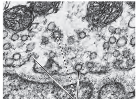
图 15.4.2: 突触小泡通过胞吐作用释放递质，并通过胞吞作用回收。左边的图像是神经肌肉接头处的冷冻断裂电子显微照片。冷冻断裂技术通过沿着脂质双层的疏水内部分裂膜来暴露膜内区域。如图 15.2.2A 所示，显示的视图是从突触间隙向上看的双层突触前膜的细胞质小叶。如图 15.2.2A 所示，右侧的传统薄层电子显微照片显示了突触前末梢、突触间隙和突触后肌膜的横截面视图 [106] 。右侧的薄层图像显示了与活动区相邻的突触小泡。 B. 突触小泡通过与细胞质膜融合（胞吐作用）释放递质。在这里，突触小泡在去极化刺激后 5 毫秒内通过快速冷冻组织而与细胞质膜融合。细胞质膜中的每个凹陷代表 1 个突触小泡的融合。在右侧的显微照片中，融合的囊泡被视为 \Omega 形结构。 C. 胞吐作用后，突触小泡膜通过胞吞作用恢复。在囊泡与突触前膜融合后约 10 秒内，形成包被凹坑。再过 10 秒后，包被的凹坑开始通过内吞作用夹断，形成包被的囊泡。这些囊泡储存原始突触囊泡的膜蛋白以及从细胞外介质捕获的分子。囊泡在末梢被回收或被运输到细胞体，膜成分在细胞体中被降解或回收（见第 7 章）。
