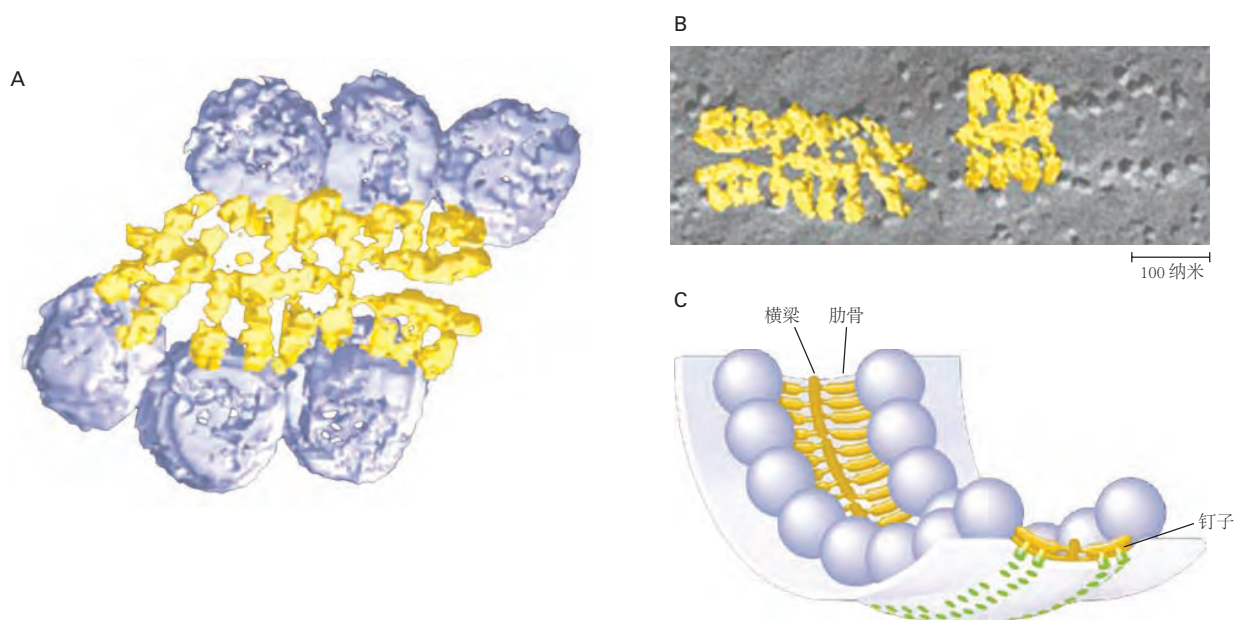
图 15.5.4: 活动区的突触小泡。图像是从电子显微镜断层扫描获得的 [118] 。A. 囊泡与活性区的丝状蛋白相连。解决了 3 种不同的丝状结构：钉子、肋骨和横梁。从囊泡突出的肋骨连接到长的水平横梁上，这些梁通过垂直销钉固定在膜上。B. 叠加在活性区膜内颗粒冻结断裂视图上的肋骨和横梁显示了肋骨如何与颗粒对齐，其中一些被认为是电压门控 \text{Ca}^{2+} 通道。C. 活动区结构的模型显示了突触小泡、钉子、肋骨和横梁之间的关系。
