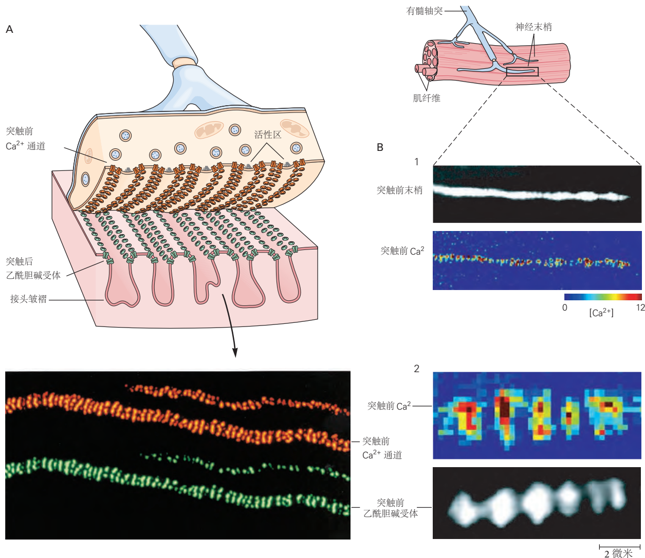
图 15.2.2: 在神经肌肉接头的突触传递过程中流入突触前神经末梢的 \text{Ca}^{2+} 集中在活动区。终板突触前末梢的 \text{Ca}^{2+} 通道集中在突触后肌膜上烟碱乙酰胆碱受体簇的对面。两幅图展示了青蛙的神经肌肉接头。A. 放大图显示了神经肌肉接头的显微解剖结构，突触前末梢被剥离。荧光图像显示了突触前 \text{Ca}^{2+} 通道（标记有与 \text{Ca}^{2+} 通道结合的德克萨斯红偶联的海洋蜗牛毒素）和突触后乙酰胆碱受体（标记有荧光标记的 \alpha -金环蛇毒素，它选择性地结合乙酰胆碱受体）。这 2 个图像通常叠加在一起，但为了清晰起见已分开。2 种探针的标记模式几乎精确对齐，表明突触前神经元的活动区与含有高浓度乙酰胆碱受体的突触后膜几乎完美对齐 [95] 。B. 突触前末梢的钙流入位于活动区。钙可以使用 \text{Ca}^{2+} 敏感的荧光染料进行可视化。1. 黑白图像显示了静息条件下充满 fura-2（细胞内 \text{Ca}^{2+} 的特异性荧光指示剂）的神经肌肉接头处的突触前末梢。染料的荧光强度随着它与 \text{Ca}^{2+} 的结合而变化。在彩色图像中，颜色编码的荧光强度变化显示细胞内 \text{Ca}^{2+} 响应单个突触前动作电位的局部热点。红色表示 \text{Ca}^{2+} 大量增加的区域；蓝色表示 \text{Ca}^{2+} 几乎没有增加的区域。沿末梢可以看到 \text{Ca}^{2+} 浓度的规则峰值，对应于 \text{Ca}^{2+} 通道在活性区的定位。2. 彩色图像显示了末梢 \text{Ca}^{2+} 水平峰值增加的高倍放大视图。相应的黑白图像显示了突触后膜中烟碱乙酰胆碱受体的荧光标记，说明了突触前 \text{Ca}^{2+} 流入区域与突触后受体区域之间的紧密空间对应关系 [96] 。
