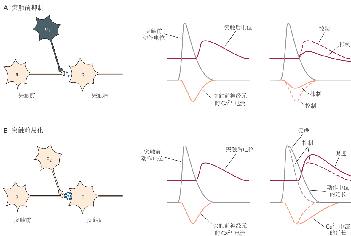
图 15.6.1: 轴-轴突触可以抑制或促进突触前细胞释放递质。A. 抑制性神经元 ( c_1 ) 在神经元 a 的轴突末梢形成突触。细胞 c_1 释放递质会激活末梢代谢受体，从而抑制末梢 Ca^{2+} 电流，减少了细胞 a 释放到细胞 b 的递质数量。细胞 a 递质释放的减少反过来又降低了细胞 b 中兴奋性突触后电位的幅度，这一过程称为突触前抑制。B. 促进神经元 ( c_2 ) 在神经元 a 的轴突末梢形成突触。细胞 c_2 释放递质会激活末梢的促代谢受体，从而降低末梢的 K^+ 电流，从而延长动作电位并增加 Ca^{2+} 流入细胞 a 。这增加了从细胞 a 到细胞 b 的递质释放，从而增加了细胞 b 中兴奋性突触后电位的大小，这一过程称为突触前促进。
