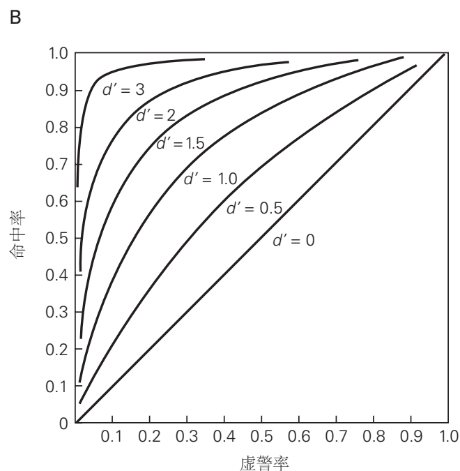
图 17.1.3: 受试者工作特征图显示试验集的结果, 每个试验都收集在如图 17.1.2A 所示的矩阵中。垂直轴绘制了命中率或概率作为水平轴上误报率或概率的函数。标记垂直轴真阳性率或灵敏度, 以及标记水平轴假阳性率或 (1 - 特异性) 也很常见。随机提供是或否响应的一组试验 (可辨别性 [ d' ] = 0) 绘制为从原点到右上角的直线。这种受试者工作特征的曲线下面积将为 0.5。一组完美的试验, 其中观察者准确地检测到每个刺激的存在并且不会被任何没有刺激的试验所愚弄 ( d' > 3 ), 将沿着左轴急剧上升, 并且曲线下面积将为 1.0。曲线下面积越来越多地被引用为单个数字的置信度度量。所示的 (理论) 曲线证明了 d' 的较高值如何导致较大的曲线下面积 [121] 。
