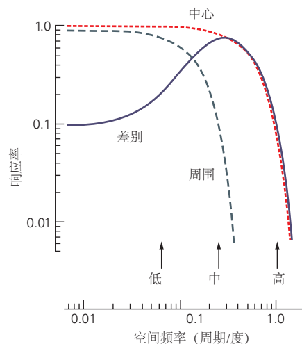
图 22.5.3: 空间对比敏感度。A. 1. 如图 22.5.4 所示，人类受试者的对比敏感度使用具有不同空间频率的光栅测量。如图所示，在每个频率下，对比度增加到检测阈值，并且该对比度值的倒数相对于空间频率绘制。这些曲线是在不同的平均强度下获得的，从顶部到底部曲线减少了 10 倍 [202] 。2. 在高强度下测量的猕猴视网膜中 P 型神经节细胞的对比敏感度。在每个空间频率下，对比度逐渐增加，直到它在神经元的放电率中产生可检测的变化。如 A-1 部分所示，绘制了该阈值对比度的倒数。左侧的孤立点标记了零空间频率下的灵敏度，这是一个空间均匀的场 [203] 。B. 用正弦光栅刺激中心环绕感受野。神经元对视网膜上不同点的光的敏感性被建模为“高斯差分”感受野，其中兴奋性中心为窄正高斯分布，抑制性周围为宽的负高斯分布。将光栅刺激的轮廓（强度与位置）与感受野的轮廓（灵敏度与位置）相乘，并在所有空间上积分，计算出特定光栅传递的刺激强度。右图显示了感受野对不同频率光栅的灵敏度。在低空间频率下，环绕声的负贡献抵消了中心的贡献，导致差异曲线下降 [204] 。
