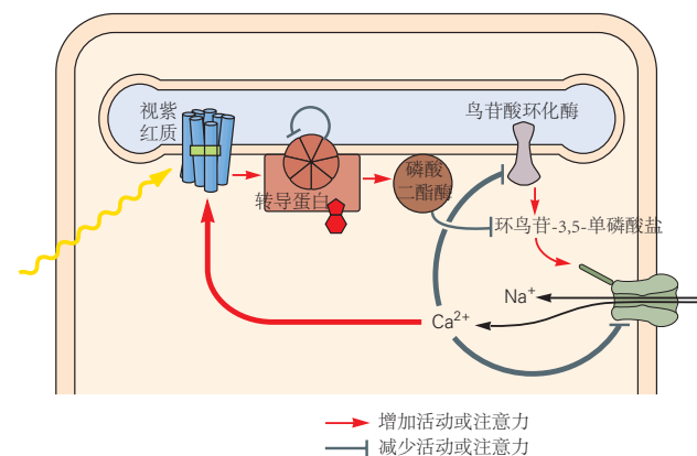
图 22.2.1: 光转导。 A. 视杆细胞对光有响应。外段视盘中的视紫红质分子吸收光子，导致细胞质膜中环鸟苷-3,5-单磷酸盐门控通道关闭。这种通道关闭使膜超极化并降低神经递质谷氨酸的释放速率 [7] 。B. 1. 光转导中的分子过程。环鸟苷-3,5-单磷酸盐由鸟苷酸环化酶从三磷酸鸟苷产生并被磷酸二酯酶水解。在黑暗中，磷酸二酯酶活性低，环鸟苷-3,5-单磷酸盐浓度高，环鸟苷-3,5-单磷酸盐门控通道开放，允许 \text{Na}^+ 和 \text{Ca}^{2+} 流入。在光线下，视紫红质通过吸收光子而被激发，然后激活转导蛋白，转导蛋白进而激活磷酸二酯酶；环鸟苷-3,5-单磷酸盐水平下降，膜通道关闭，更少的 \text{Na}^+ 和 \text{Ca}^{2+} 进入细胞。转导酶均位于内膜圆盘，可溶性配体环鸟苷-3,5-单磷酸盐作为细胞质膜的信使。2. \text{Ca}^{2+} 在光转导响应级联中具有负反馈作用。光对网络的刺激导致环鸟苷-3,5-单磷酸盐门控通道的关闭。这导致细胞内 \text{Ca}^{2+} 浓度下降。因为 \text{Ca}^{2+} 调节至少 3 个级联组分的功能（视紫红质、鸟苷酸环化酶和环鸟苷-3,5-单磷酸盐门控通道） \text{Ca}^{2+} 的下降抵消了光引起的激发。C. 灵长类视杆细胞和视锥细胞对强度增加的短暂闪光的电压响应。迹线上的数字越高表示光照强度越大（并非所有迹线都已标记）。对于昏暗的闪光，响应幅度随强度线性增加。在高强度下，受体饱和并在闪光后的一段时间内稳定地保持超极化；这会导致我们在明亮的闪光后看到的残像。请注意，对于更亮的闪光，响应峰值更早，并且视锥细胞的响应速度比视杆细胞快 [196] 。
