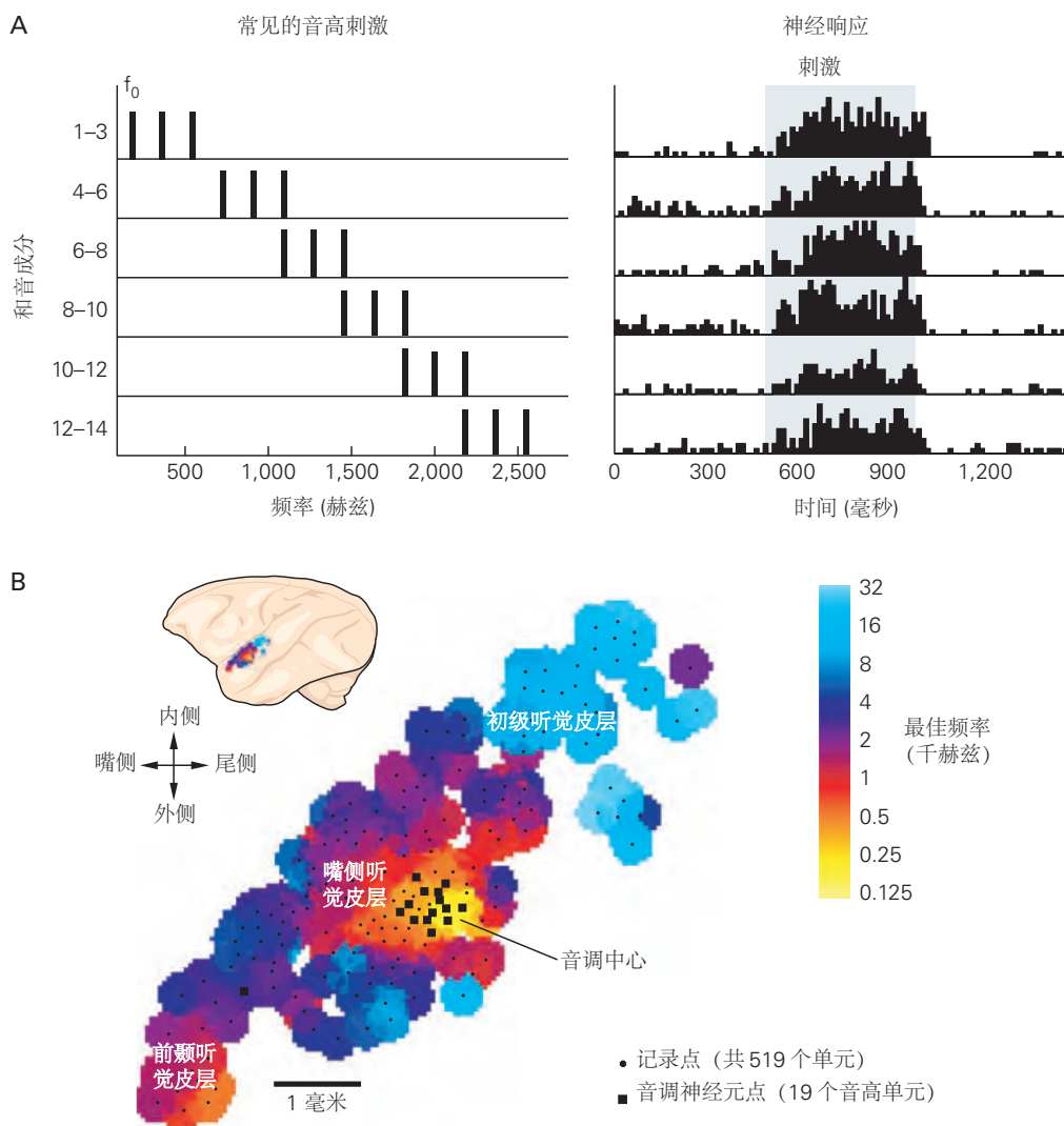
图 28.6.2: 音调由灵长类动物听觉皮层中的专门神经元编码。A. 从狒猴听觉皮层记录的音高选择性神经元的例子。左图：一系列共享相同基频 ( f_0 ) 的谐波刺激频谱。右图：神经元对刺激响应的周围刺激时间直方图 (阴影区域表示的刺激持续时间) [261] 。B. 狒猴听觉皮层的解剖组织和音高中心的位置。上图：狒猴大脑的侧视图。底部：一只狒猴典型的左听觉皮层音调映射。音高选择性神经元 (黑色方块) 聚集在初级听觉皮层和嘴侧听觉皮层之间的低频边界附近。频率反转表示“初级听觉皮层/嘴侧听觉皮层”和“嘴侧听觉皮层/前颞听觉皮层”之间的边界 [261] 。
