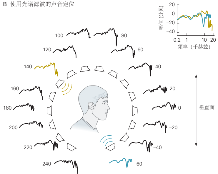
B 使用光谱滤波的声音定位
