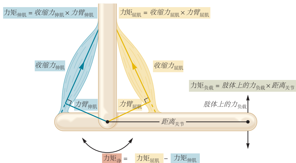
图 31.3.1: 肌肉扭矩在关节周围的运动范围内变化。肌肉对关节的扭矩是其收缩力 (牛) 及其相对于关节的力臂 (d) 的乘积。力臂是从肌肉拉力线到关节旋转中心的最短垂直距离。由于关节旋转时力臂会发生变化, 因此肌肉扭矩会随着关节周围的角位移而变化。决定机械动作的关节净力矩是相对肌肉施加的扭矩的差异, 例如伸肌和屈肌。类似地, 施加到肢体上的力将围绕关节施加扭矩, 该扭矩取决于施加到肢体上的力及其与关节的距离。
