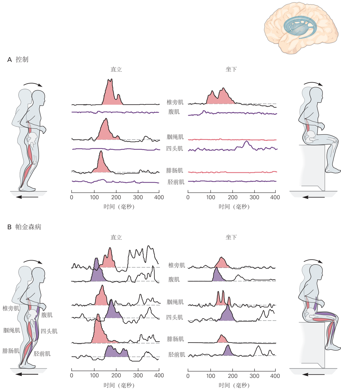
图 36.5.3: 基底神经节对于适应初始条件突然变化的姿势响应很重要 [360] 。A. 当正常受试者从直立姿势转换为坐姿时，他会立即改变对支撑平台向后移动的响应。坐着时对运动的姿势响应不涉及腿部肌肉（腓肠肌和腿筋），但会激活椎旁肌，并且比站立时对运动的响应延迟更短。B. 帕金森病患者在从站立转为坐姿后的第一次试验中没有抑制腿部肌肉响应。该受试者的姿势响应对于 2 个初始位置都相似：拮抗肌（紫色）与激动肌（粉红色）一起被激活。
