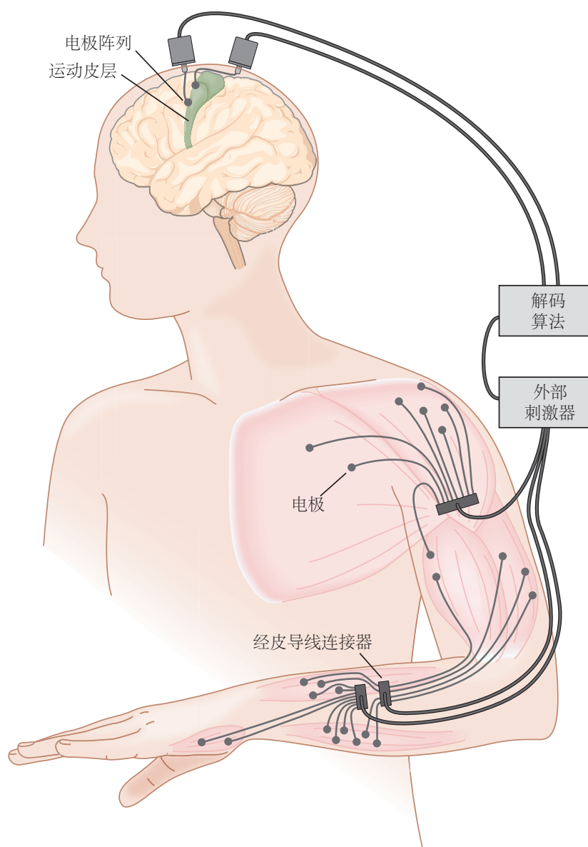
图 39.3.5: 运动脑机接口可以使用连续解码器和功能性电刺激来控制瘫痪手臂的肌肉。将运动皮层中记录的神经活动解码为控制三角肌、胸大肌、二头肌、三头肌、前臂和手部肌肉刺激的命令信号。这使得皮层能够控制整个手臂的运动和抓握。肌肉刺激是通过经皮肌肉内细线电极进行的 [380] 。
