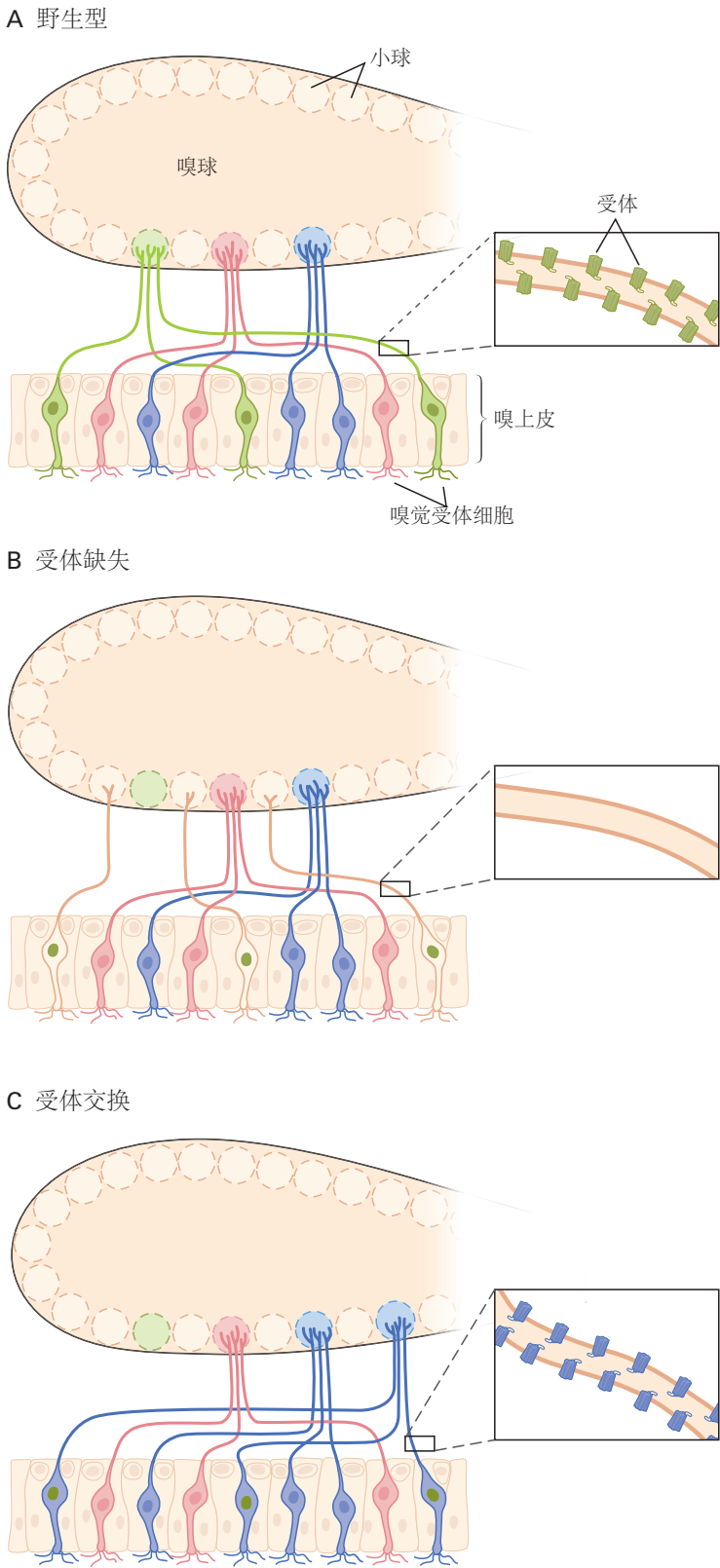
图 48.1.3: 气味受体影响感觉轴突靶向嗅球中离散球状体 [429] 。A. 每个嗅觉受体神经元表达大约 1 千种可能的气味受体中的一种。表达相同受体的神经元稀疏地分布在整个鼻子的嗅觉上皮细胞中。这些神经元的轴突与嗅球中单个小球中的目标神经元形成突触。B. 在气味受体基因被删除的小鼠突变体中，本应表达该基因的感觉神经元将其轴突发送到其他小球，部分原因是这些神经元现在表达了其他受体。C. 当一组感觉神经元中的一个气味受体基因取代另一个时，它们的轴突投射不正常。
